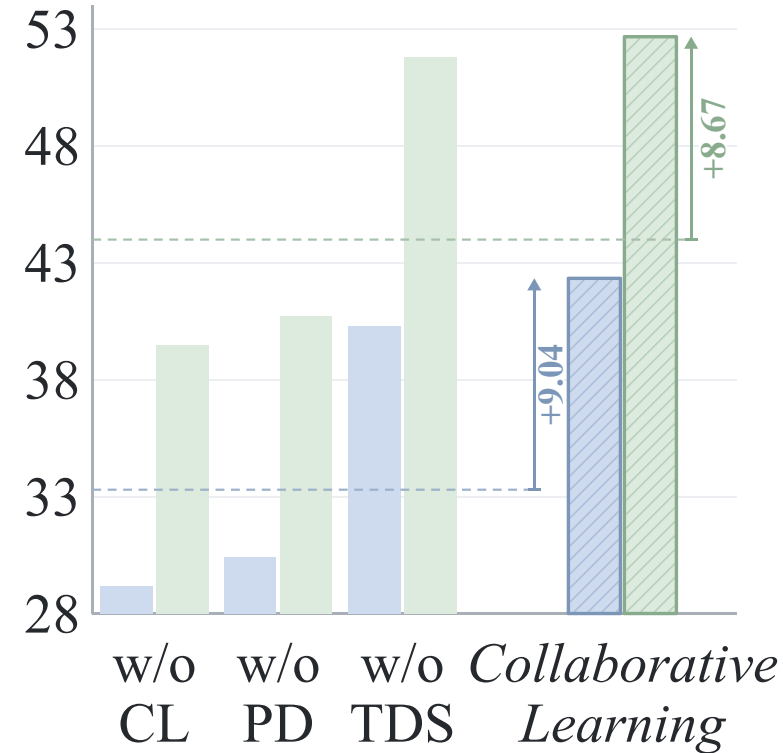
MuSiQue
