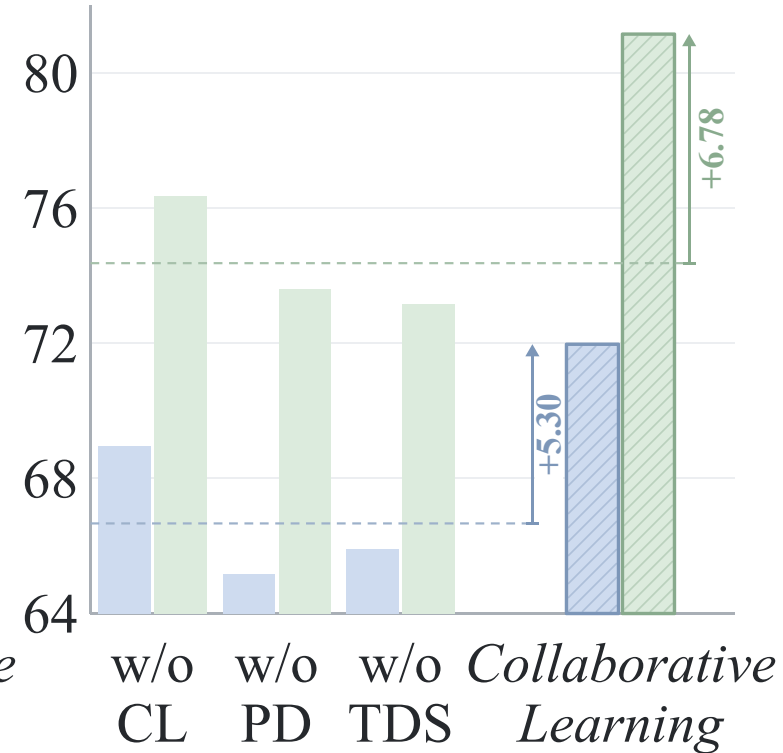
GSM-Hard
