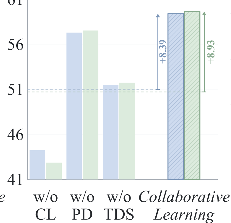
MultiPL-E
