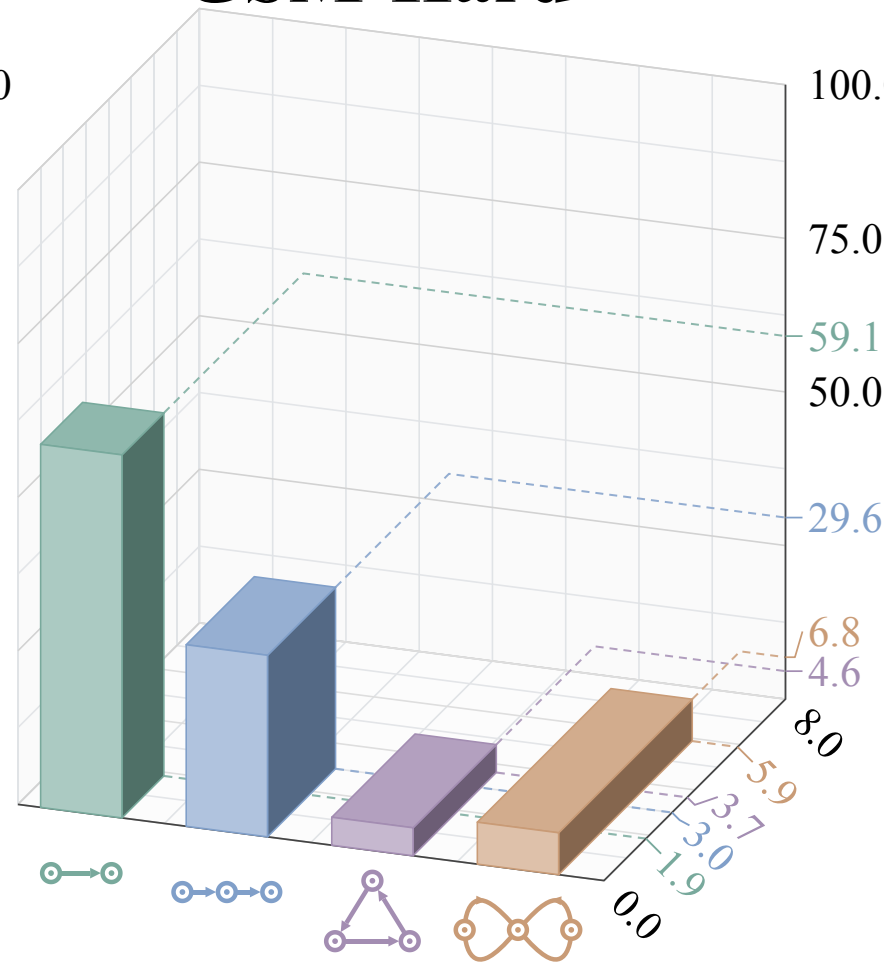
GSM-Hard
