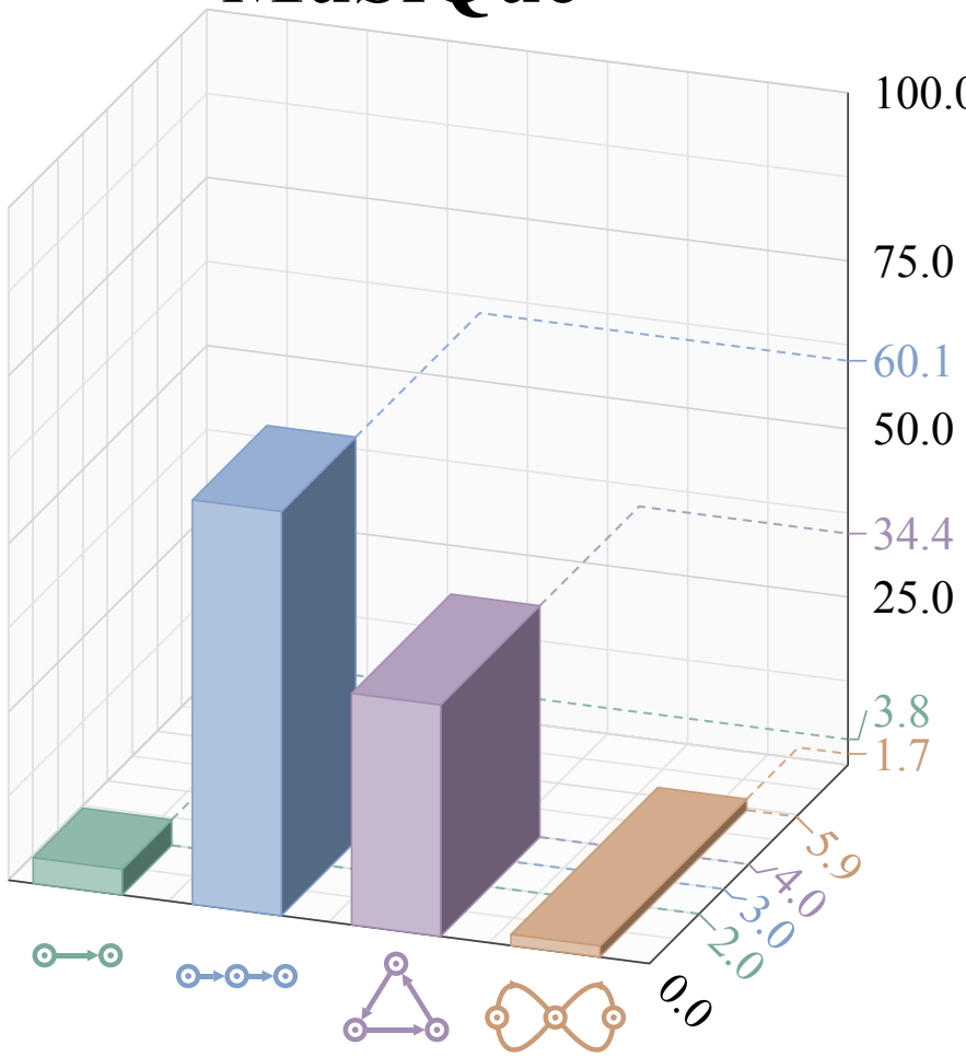
MuSiQue
