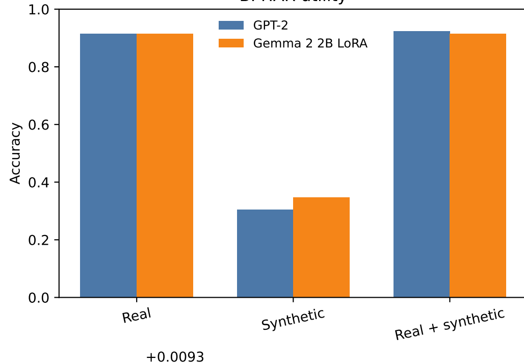
B. HAR utility
