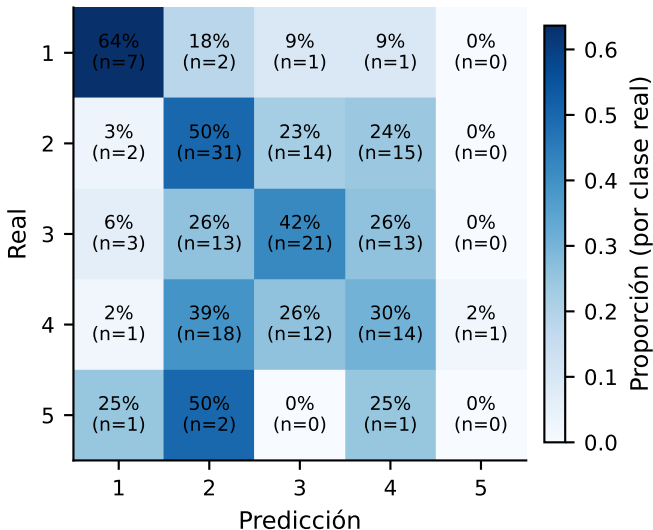
Matriz de confusión normalizada
