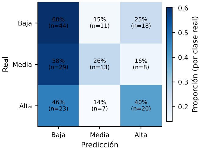
Matriz de confusión normalizada
