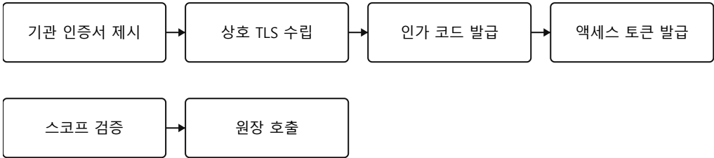
사용자 계좌 접근 인증 흐름
