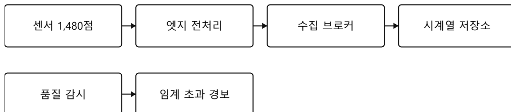
그림 2 센서에서 경고까지의 처리 흐름
