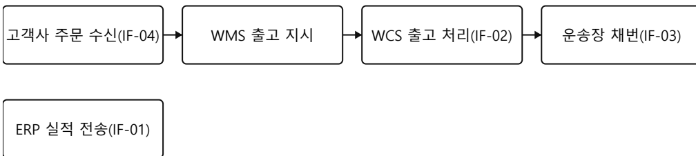
그림 1 주문 수신부터 실적 전송까지의 연계 흐름
