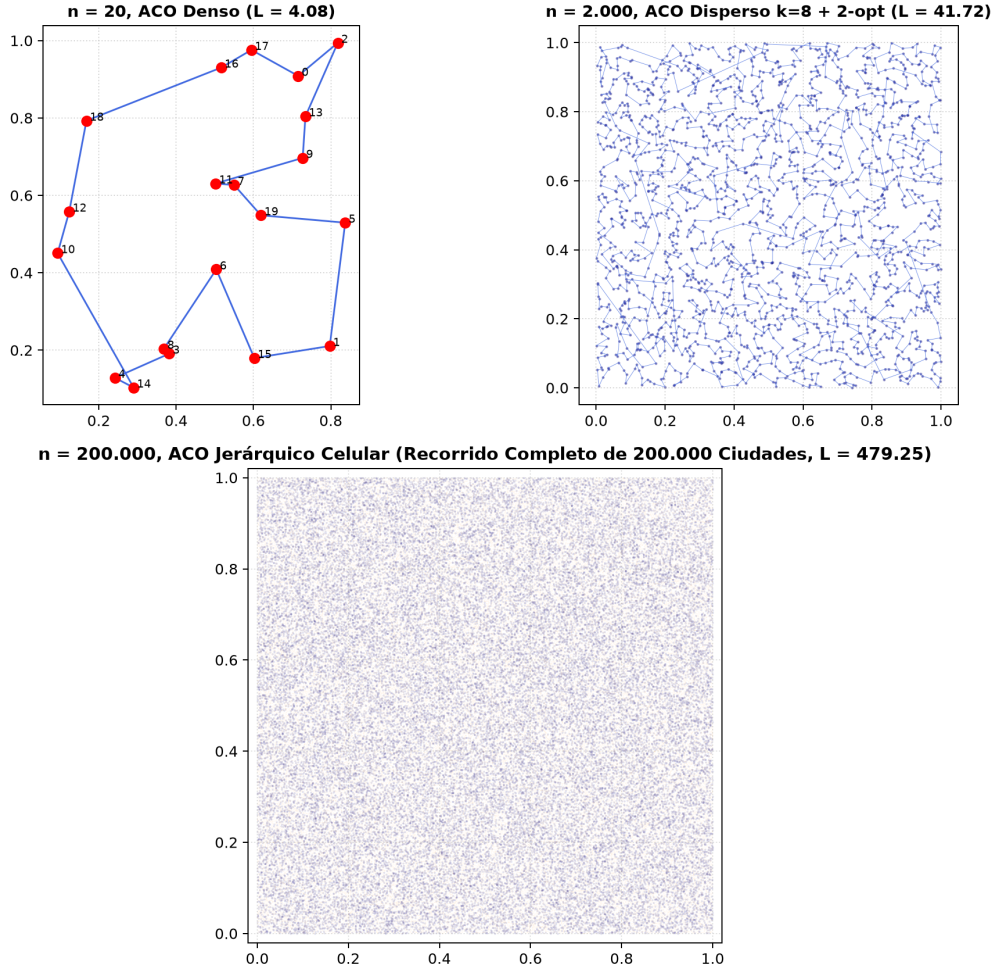
Figura 3: Visualización espacial de los circuitos: N = 20 (régimen denso) y N = 2,000 (disperso k -NN + 2-opt) en el panel superior, y N = 200,000 en la sección inferior ilustrando el recorrido hamiltoniano completo de las 200.000 ciudades ( L = 479.25 ).
