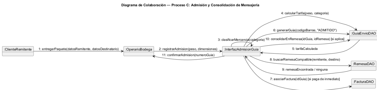
Figure 6: Diagrama de colaboración — Proceso C: Admisión y Consolidación de Mensajería
