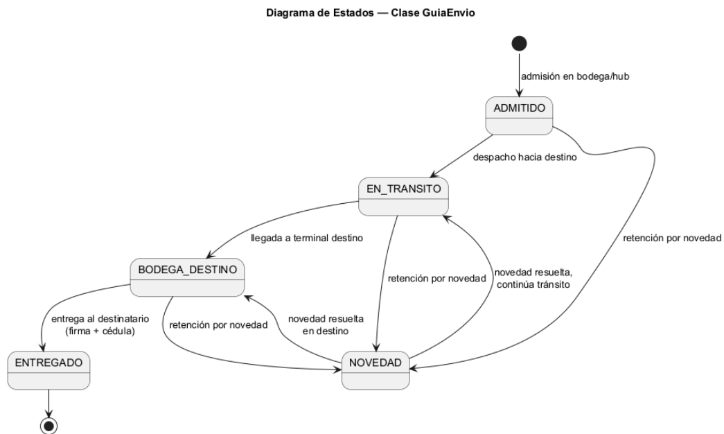
Figure 3: Diagrama de estados — Clase GuiaEnvio
