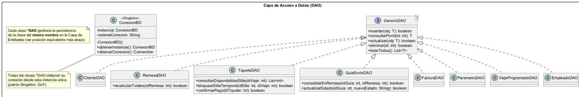
Diagrama de Clases DAO — Venta de Tiquetes y Mensajería (Copetran)
