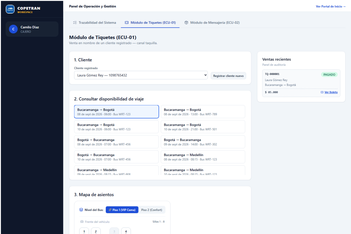
Figure 18: Módulo de Tiquetes — mapa de asientos interactivo (RF01, RF03)
