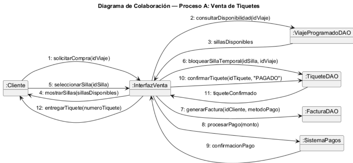
Figure 5: Diagrama de colaboración — Proceso A: Venta de Tiquetes
