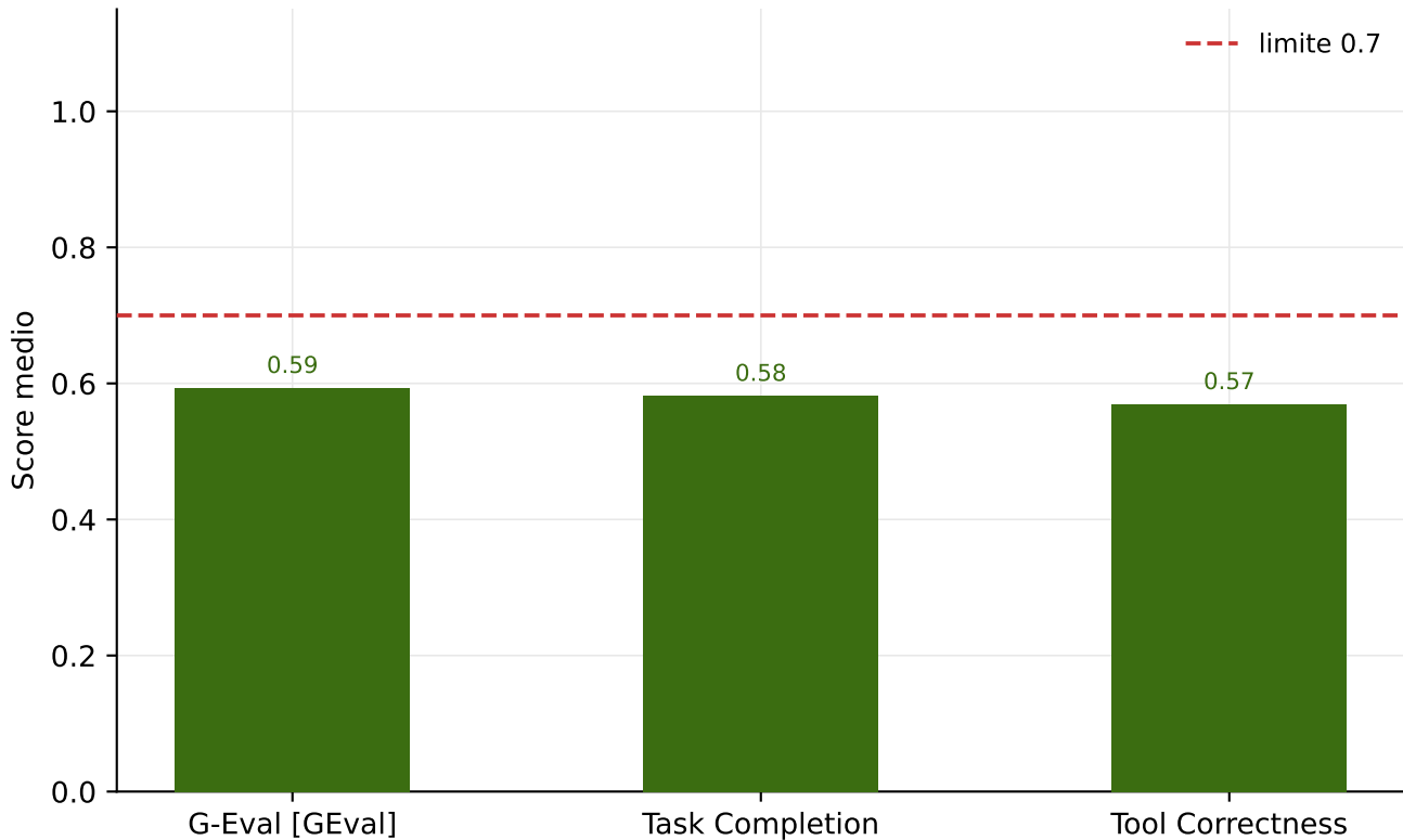
Score medio por metrica - DeepSeek-V4-Pro
