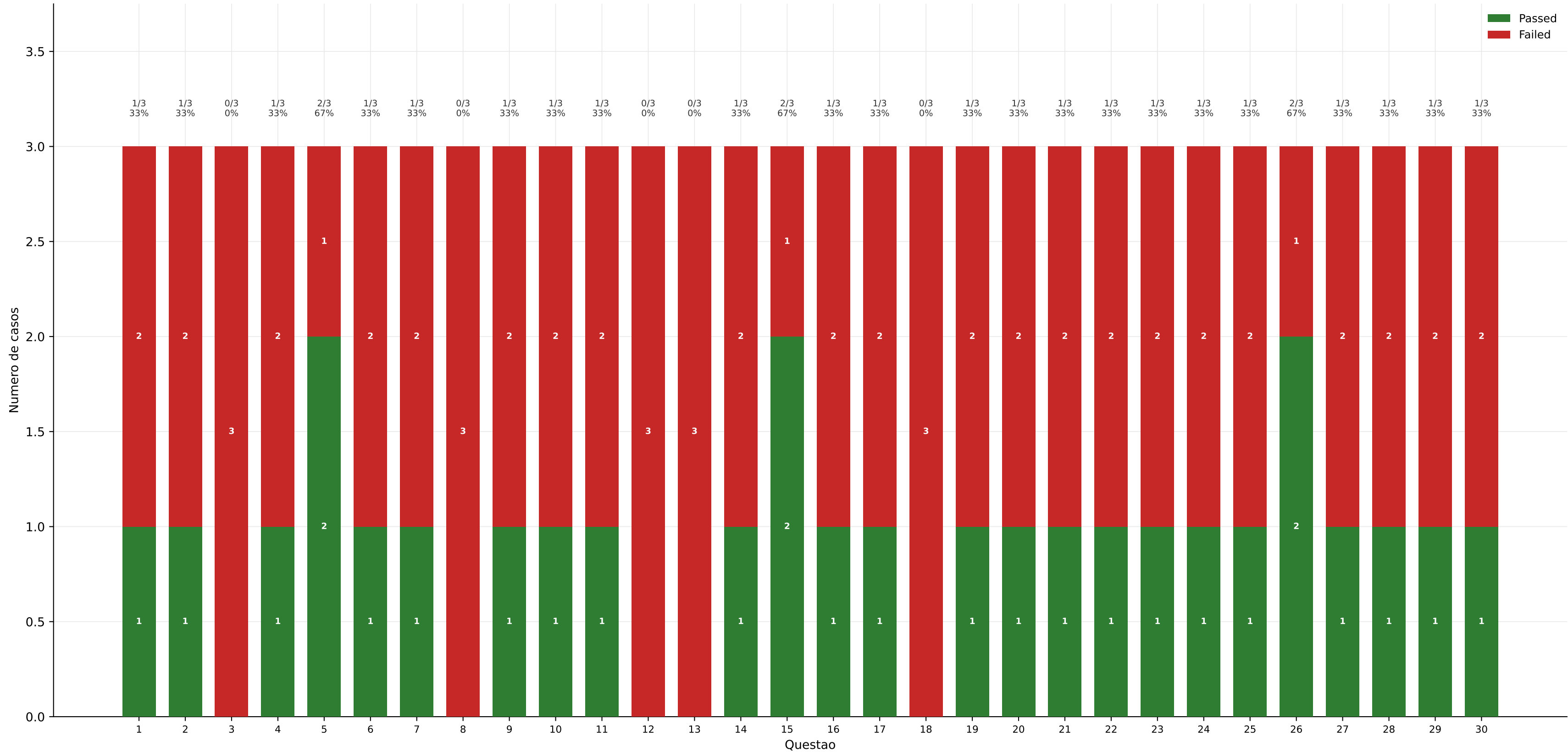
Passed vs failed por questao - MiniMax-M3
