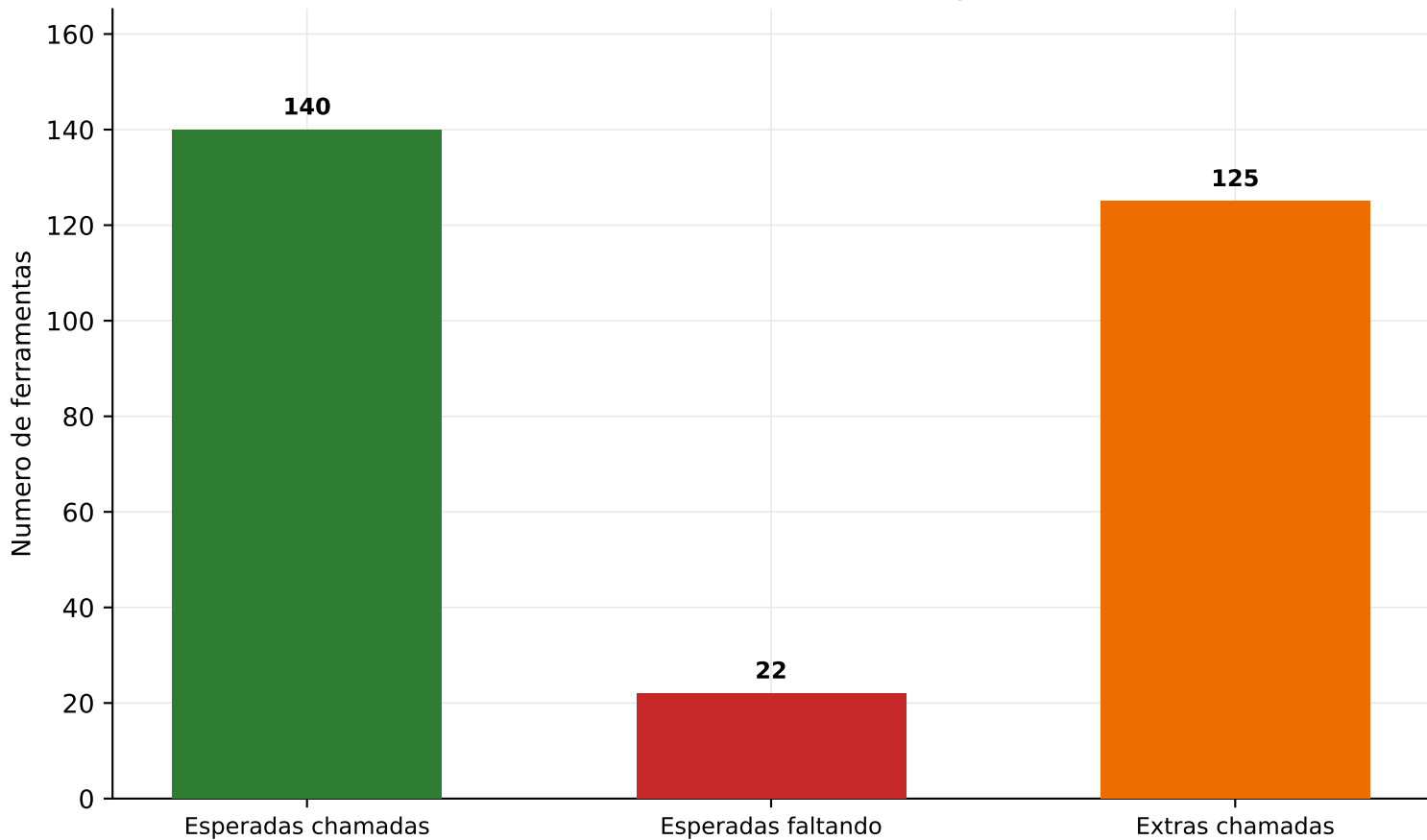
Resumo de uso de ferramentas - DeepSeek-V4-Pro
