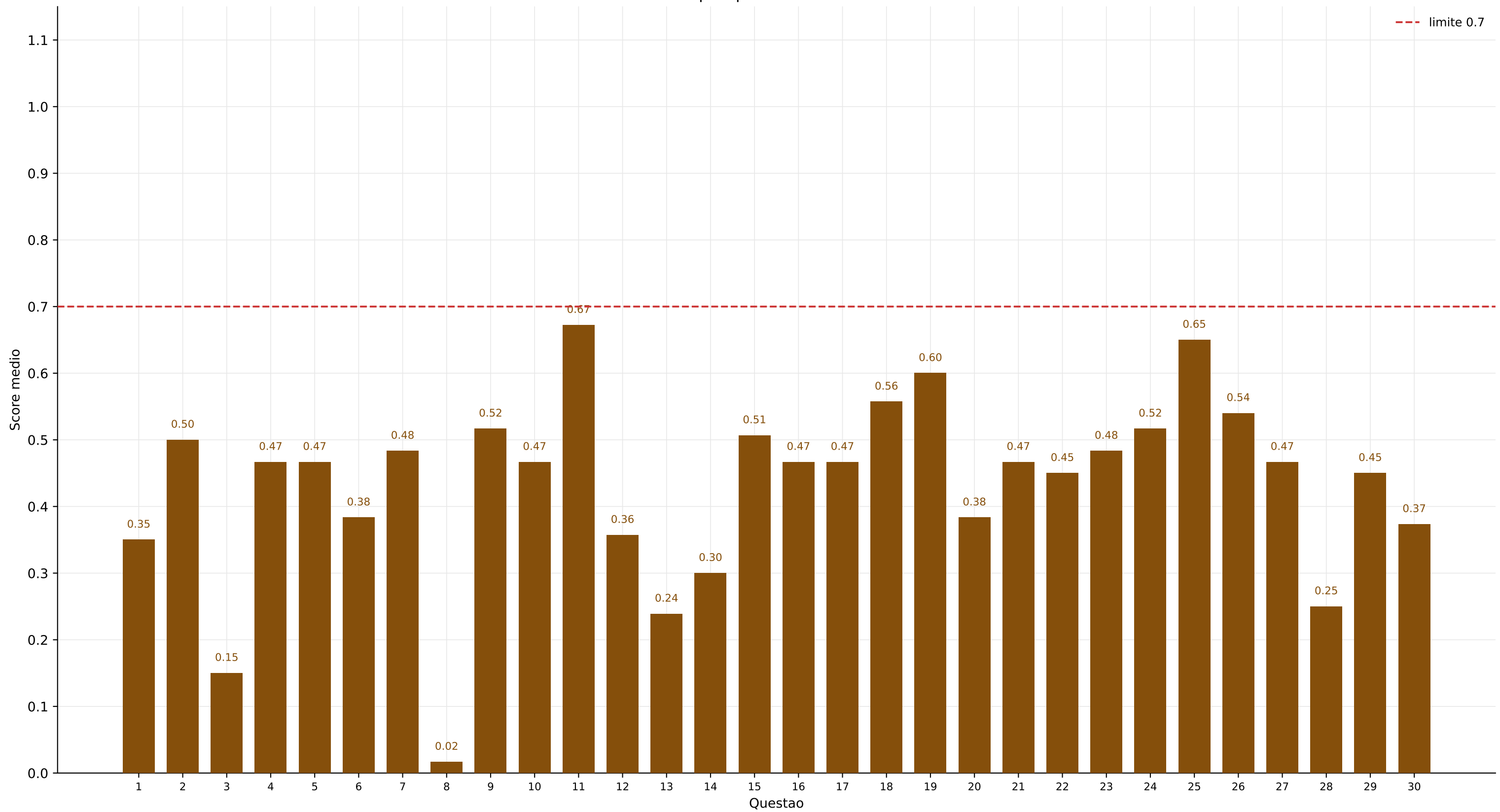
Score por questao - MiniMax-M3
