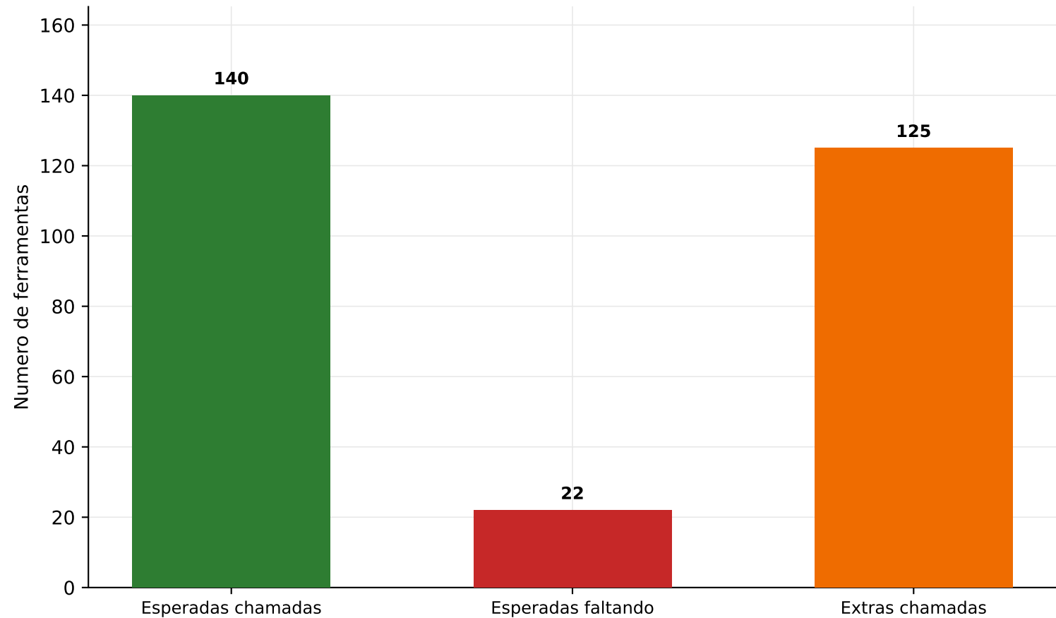
Resumo de uso de ferramentas - Gemini-3.1-Pro-Preview
