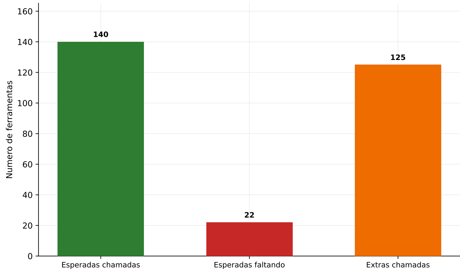
Resumo de uso de ferramentas - MiniMax-M3
