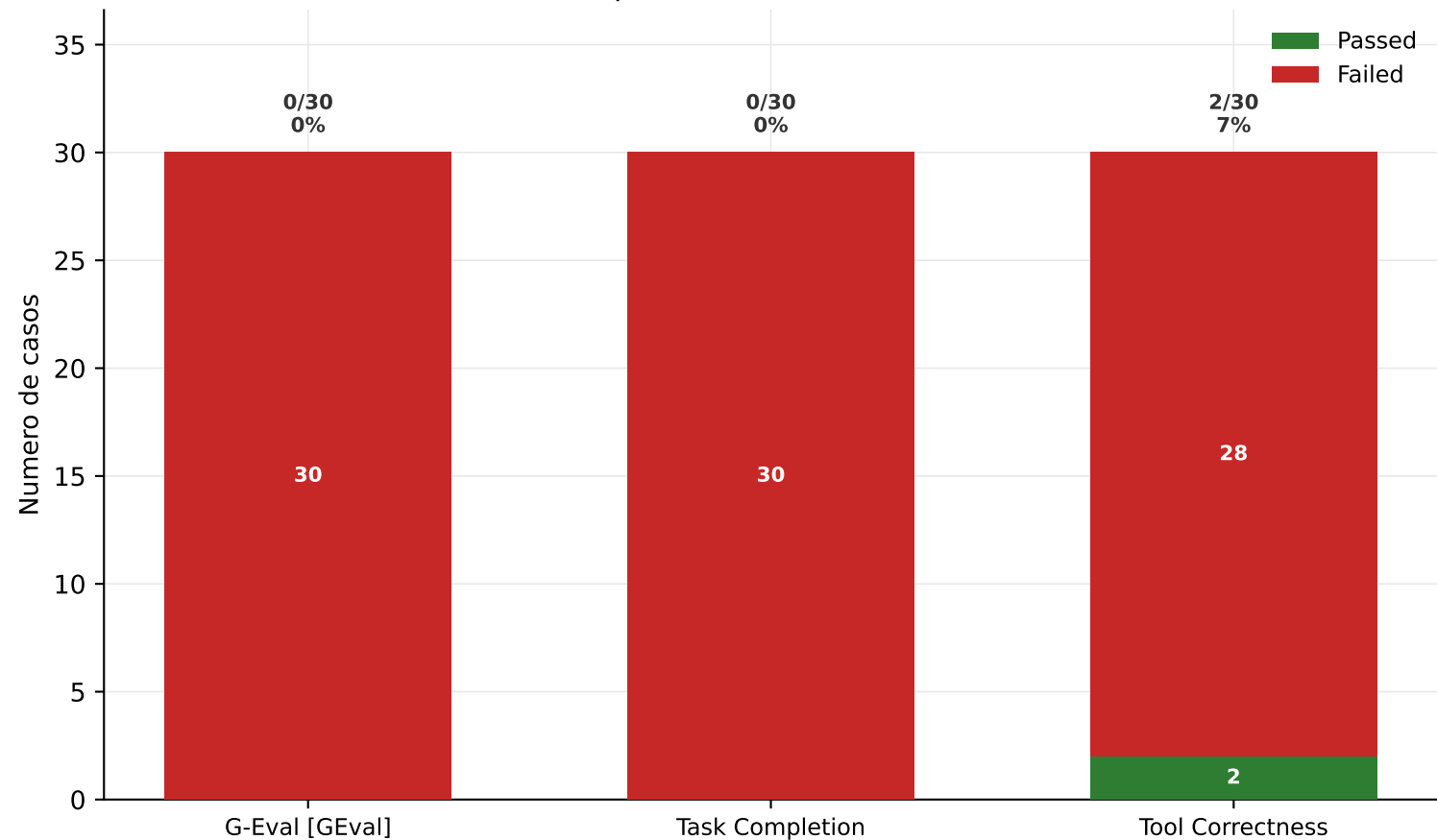
Passed vs failed por metrica - Gemini-3.1-Pro-Preview
