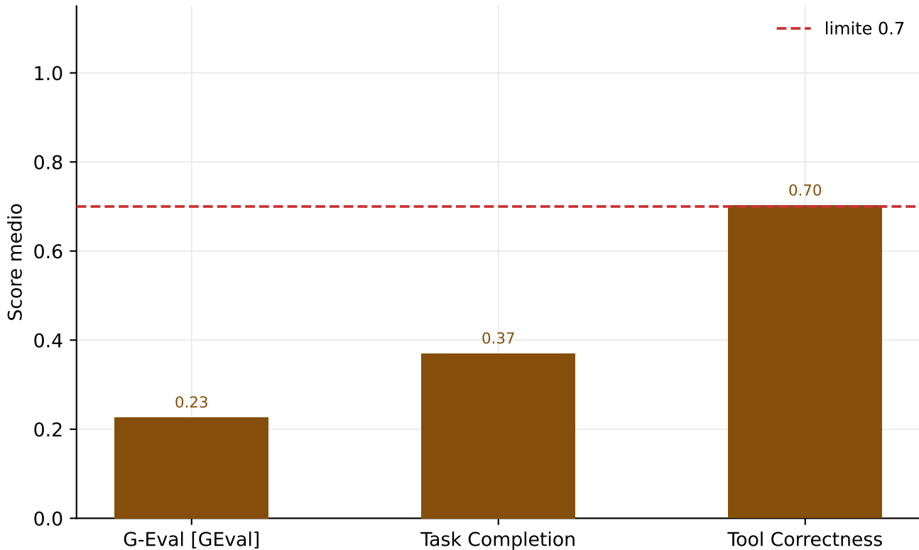
Score medio por metrica - MiniMax-M3
