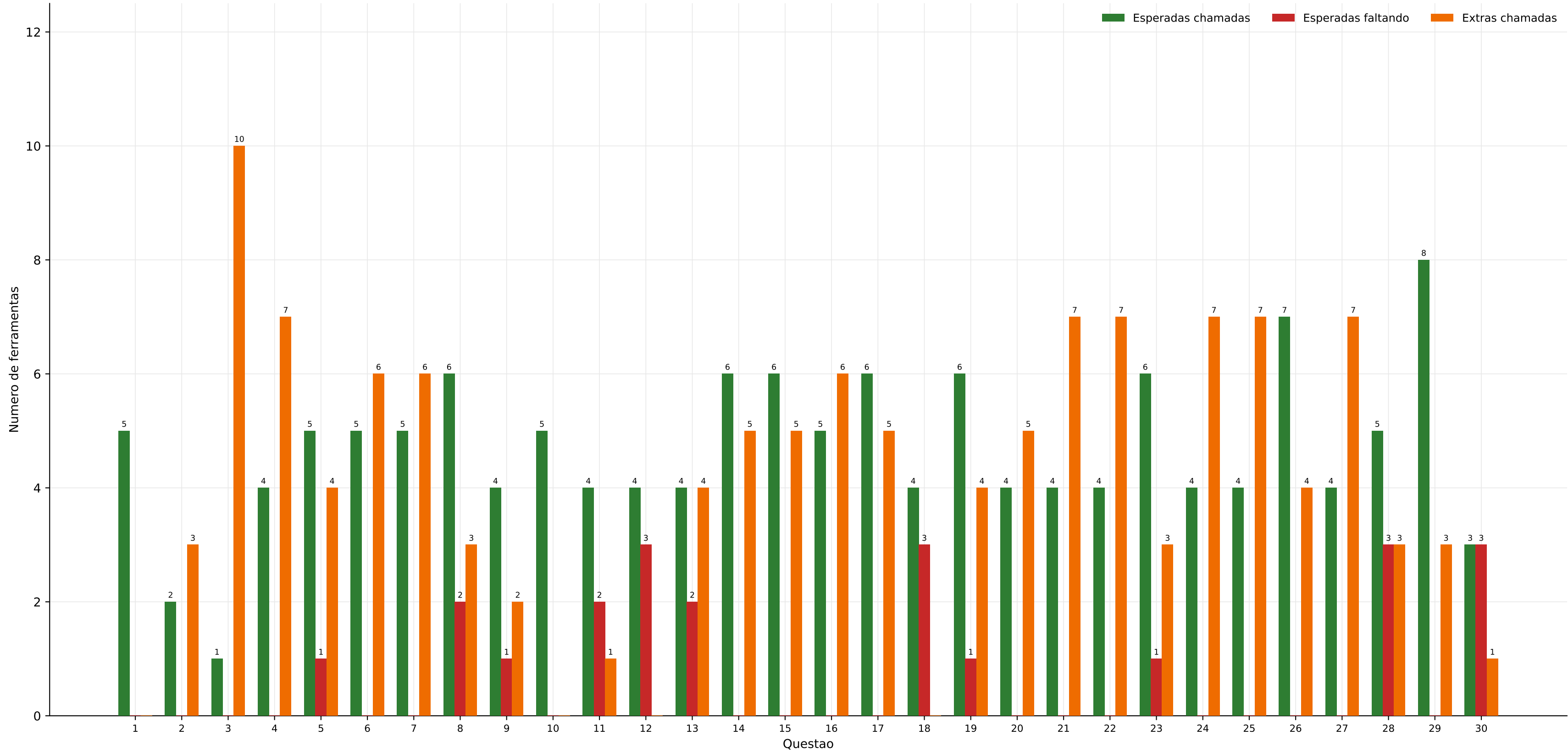
Uso de ferramentas por questao - Gemini-3.1-Pro-Preview
