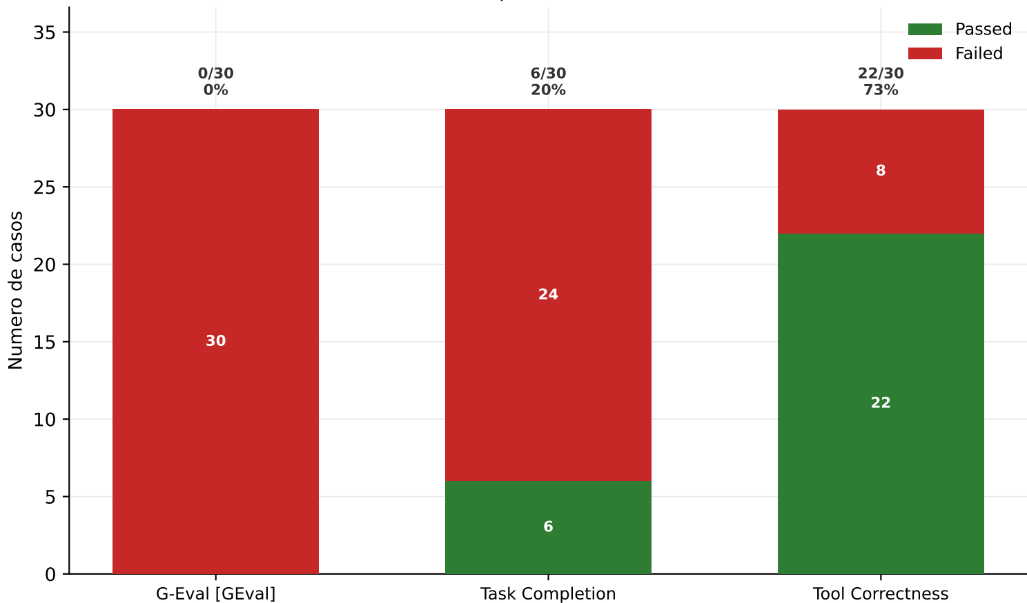
Passed vs failed por metrica - MiniMax-M3
