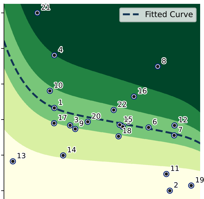
CodeXGLUE-COC
