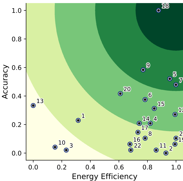
LiveCodeBench-COC
