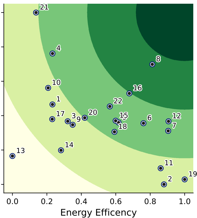
CodeXGLUE-COC
