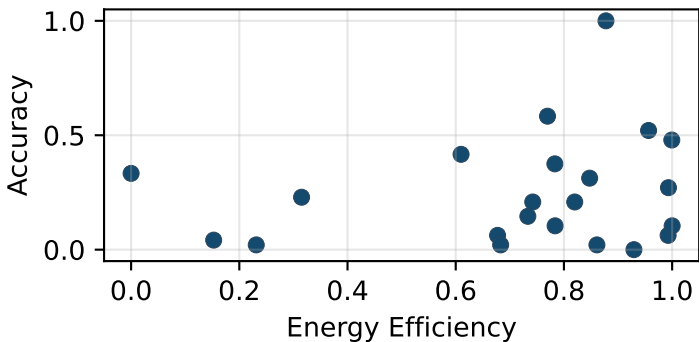
Code2Text
