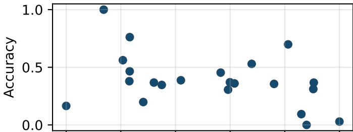
LiveCodeBench
