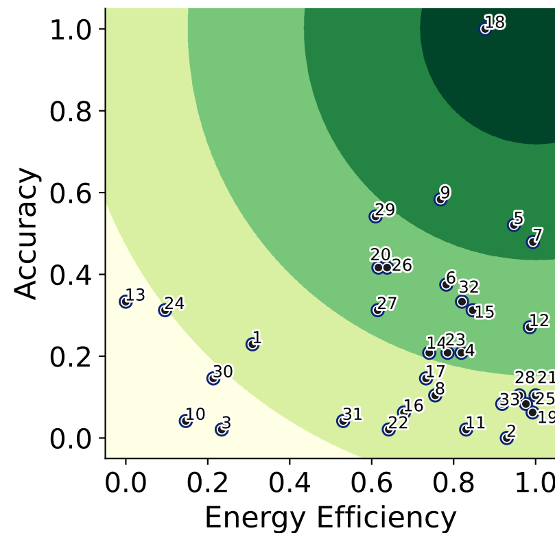
LiveCodeBench-CIRC
