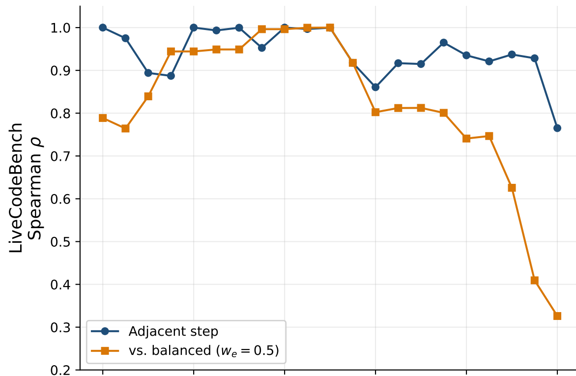
OTER
