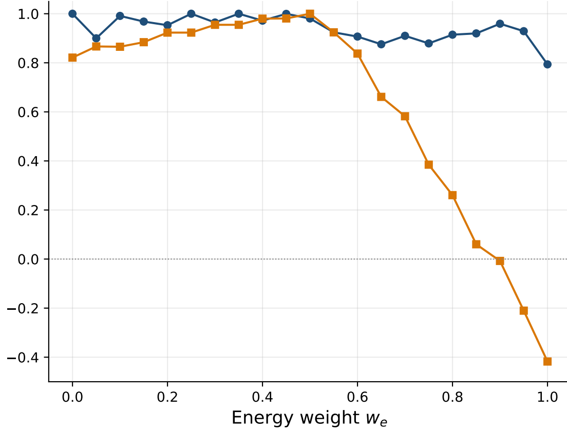
CodeXGLUE
