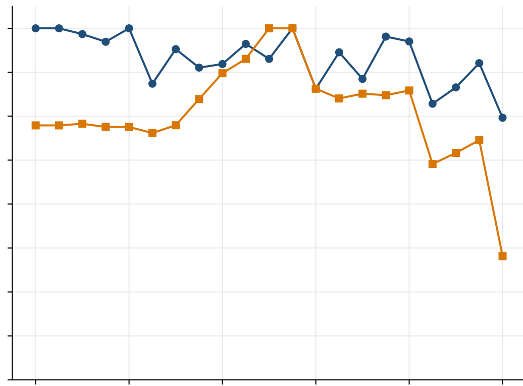
CIRC
