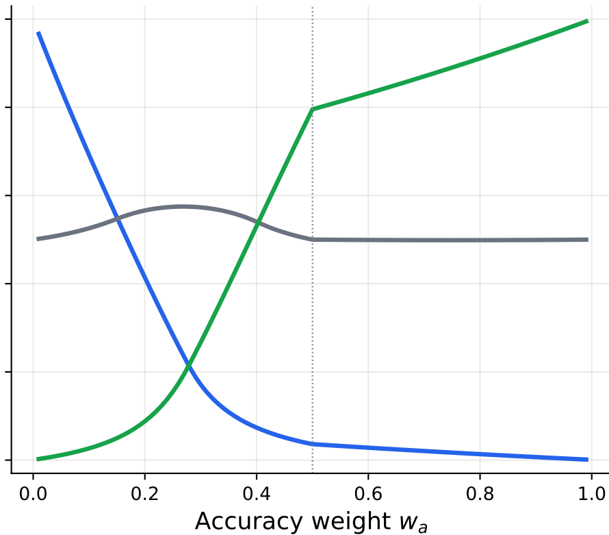
OTER · CodeXGLUE
