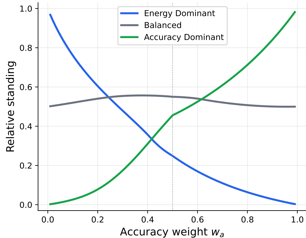
OTER · LiveCodeBench
