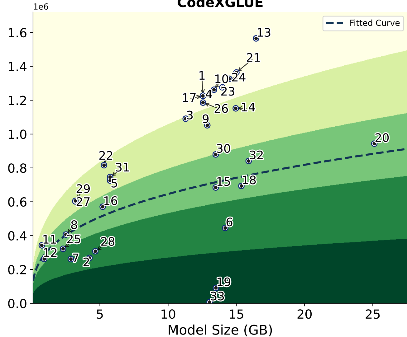
CodeXGLUE
