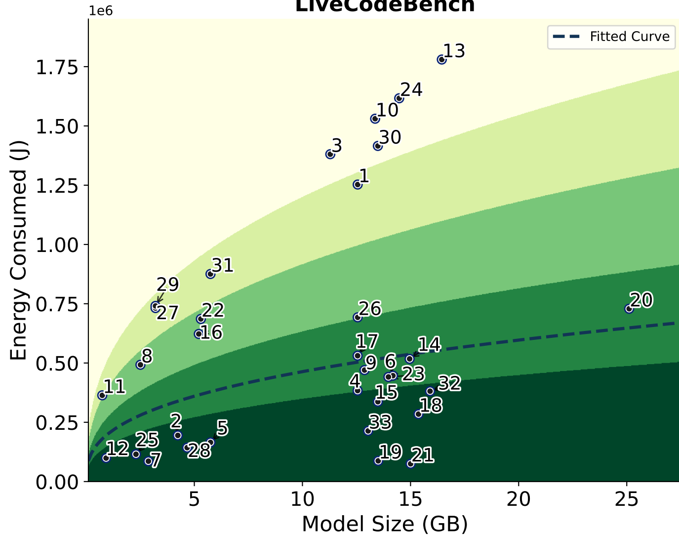
LiveCodeBench
