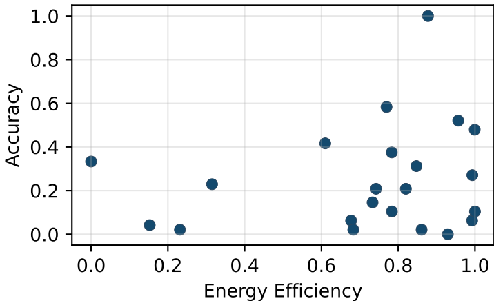
Code2Text
