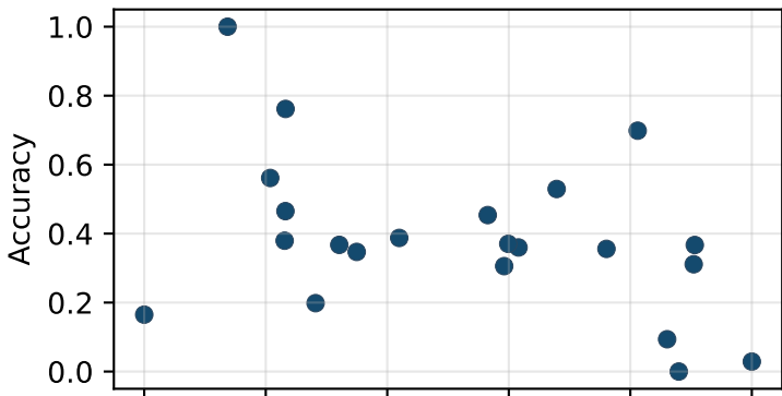
LiveCodeBench
