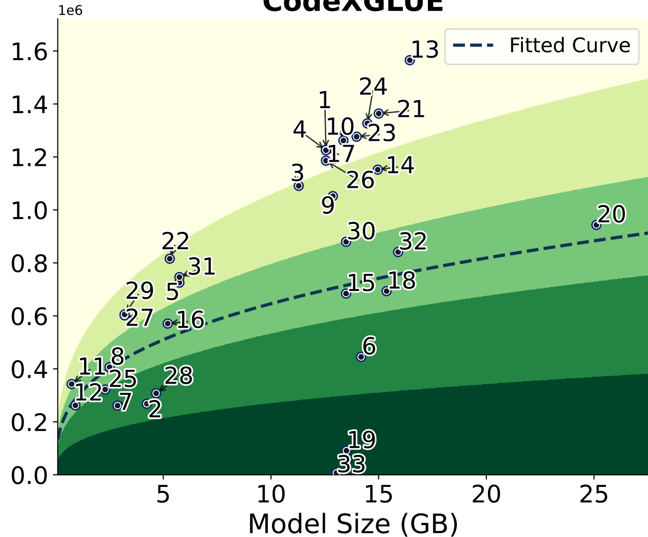
CodeXGLUE
