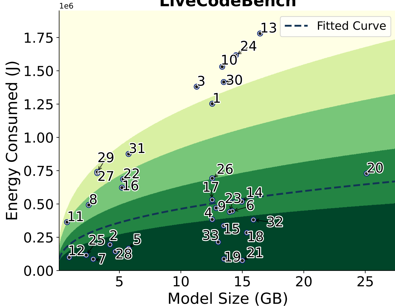
LiveCodeBench
