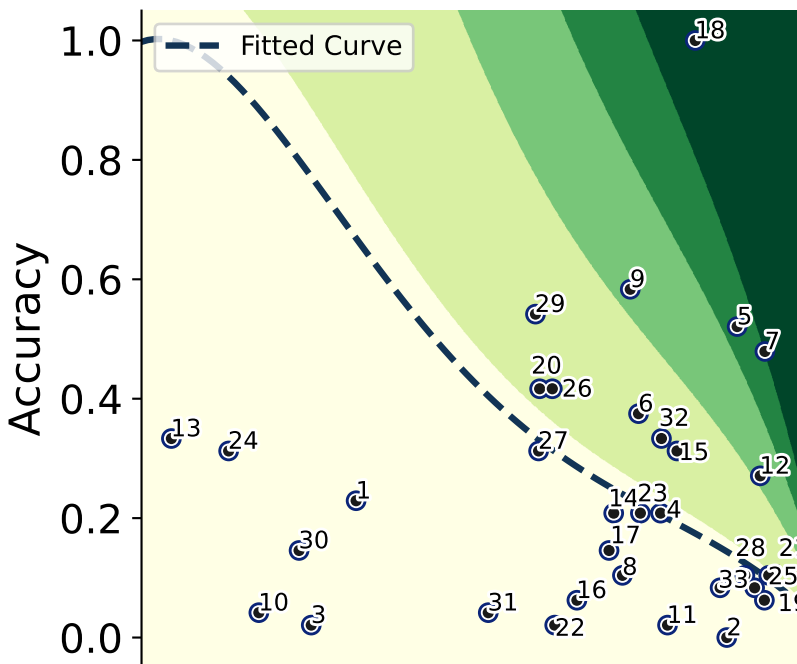
LiveCodeBench-CIRC
