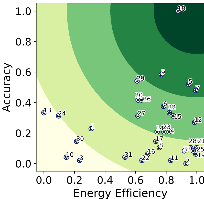
LiveCodeBench-CIRC
