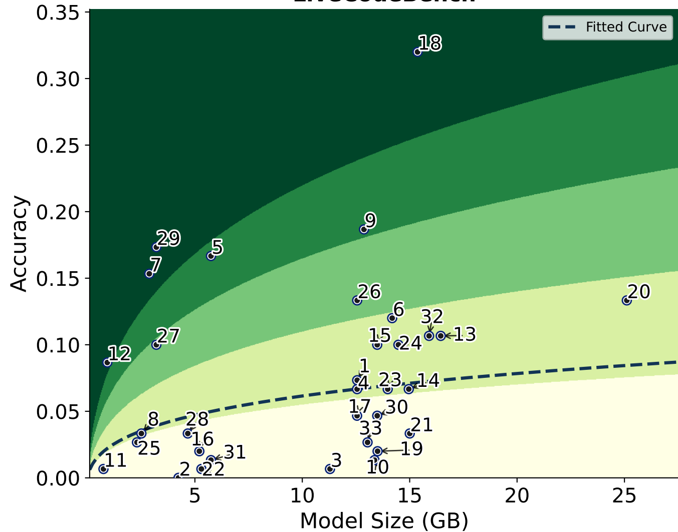
LiveCodeBench
