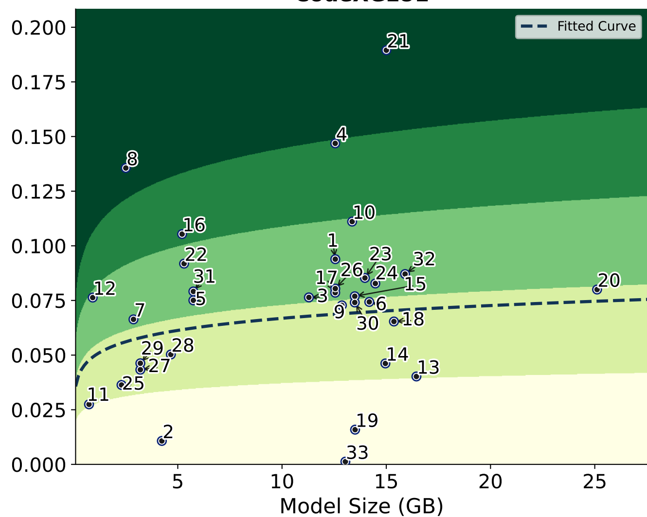
CodeXGLUE
