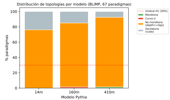
Figure 2: Distribución de topologías por modelo Pythia con criterio robusto (profundidad \geq 5 pp). La línea roja indica el umbral H1 (30%).
