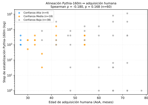
Figure 3: Scatter entre el paso de estabilización de Pythia-160M y la AoA humana. Color indica confianza del mapeo. \rho = -0,180 , p = 0,168 , n = 60 .
