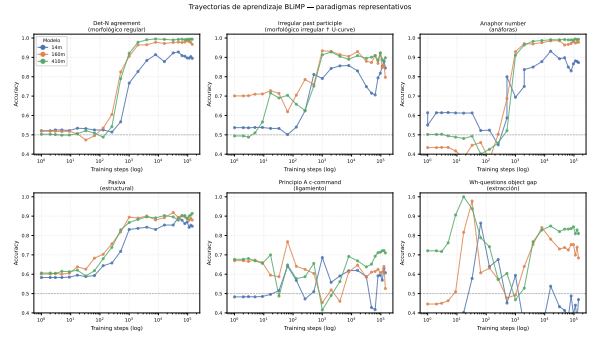
Figure 1: Trayectorias de accuracy BLiMP para seis paradigmas representativos (eje X: pasos de entrenamiento en escala log; eje Y: accuracy de pares mínimos; línea punteada: azar = 0.5).
