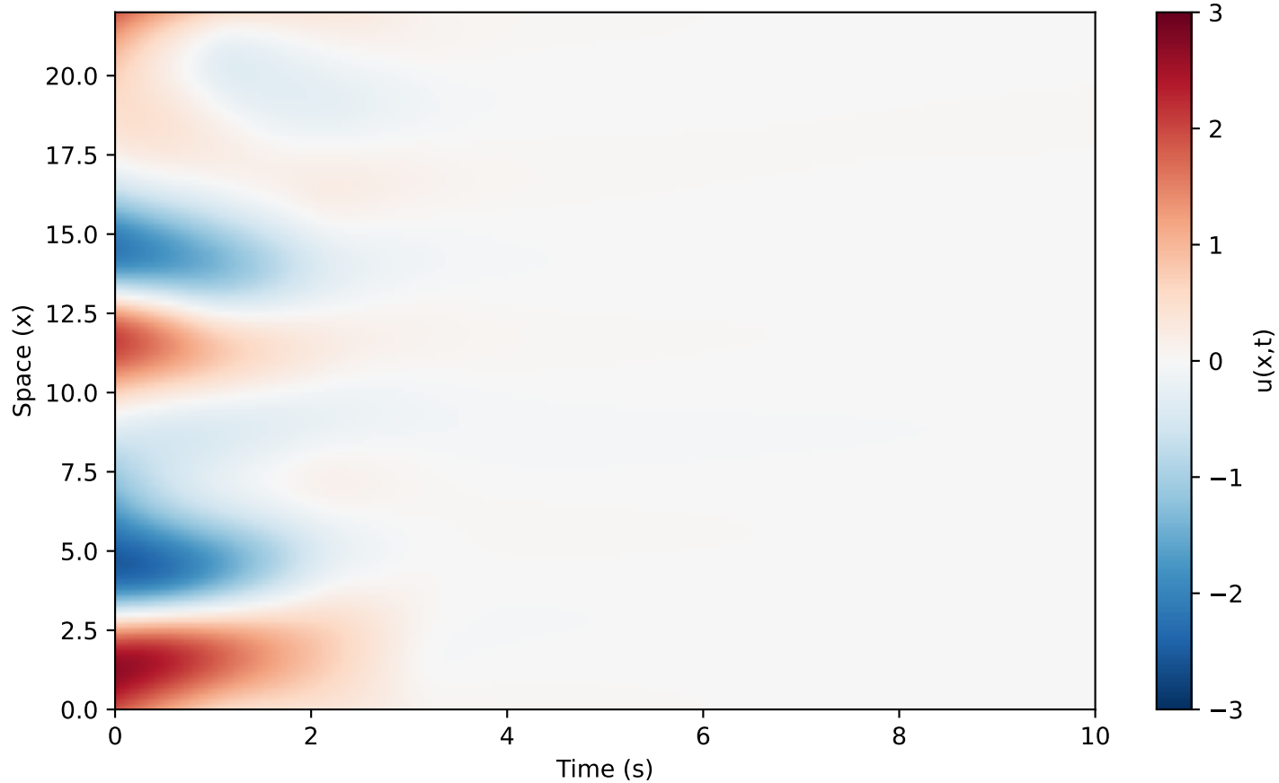
Controlled State: MAPPO
