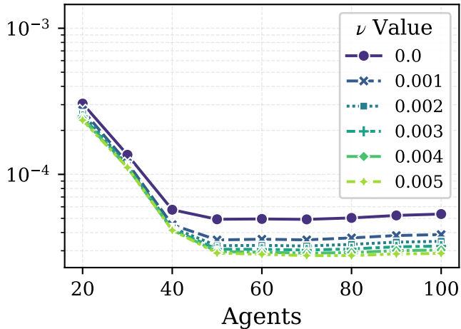
Final Tracking Error (MSE)
