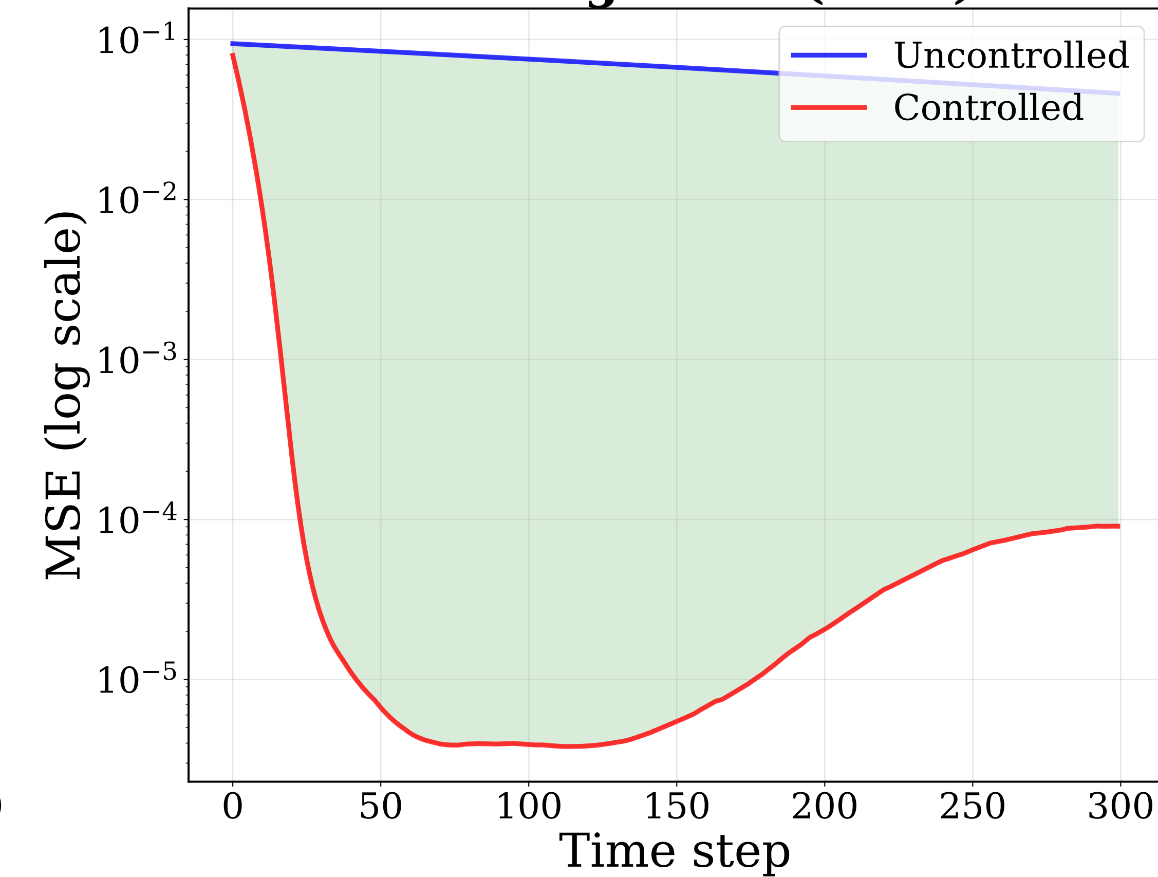
Tracking Error (MSE)
