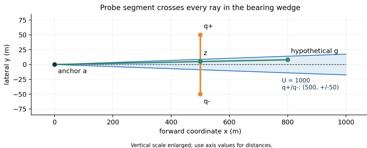
图 18: 成对测点横跨角楔，远端候选源与正锚点的连线穿过探测线段
