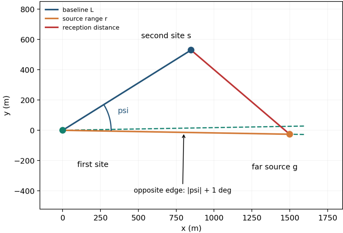
图 11: 首站、第二站及角楔另一侧的远端源：两条射线的夹角为偏角加 1 度
