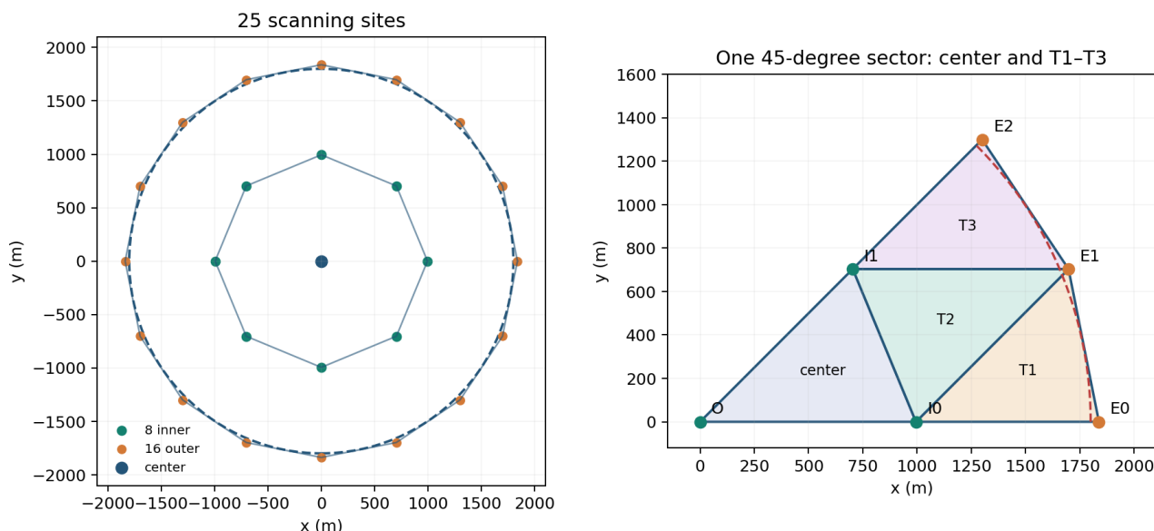
图 17: Q4 的 25 个站点，以及一个 45 度扇区的四个小三角形
