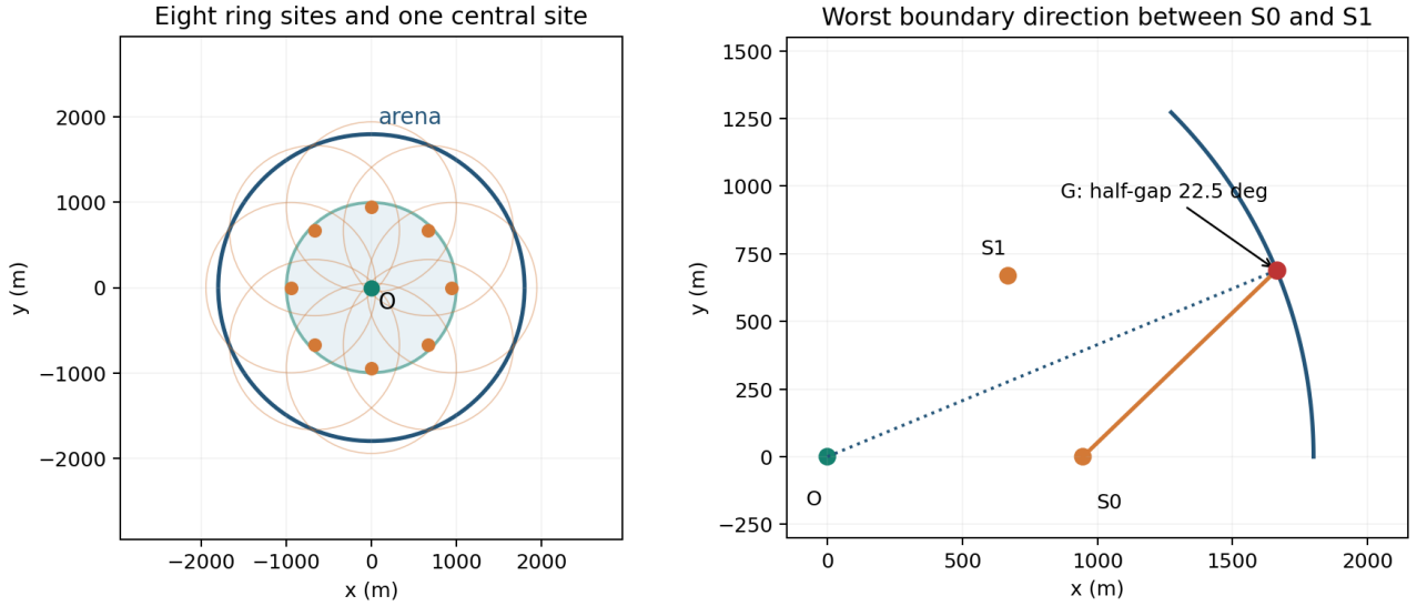
图 13: 图 5.2 Q3 九站覆盖：中心站、八个环站与 22.5° 的最大方位差
