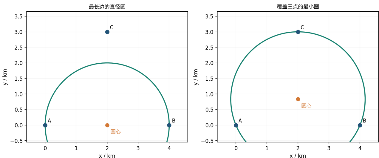
图 2: 最远点对的直径圆未覆盖第三点；右图的最小包围圆覆盖三点
