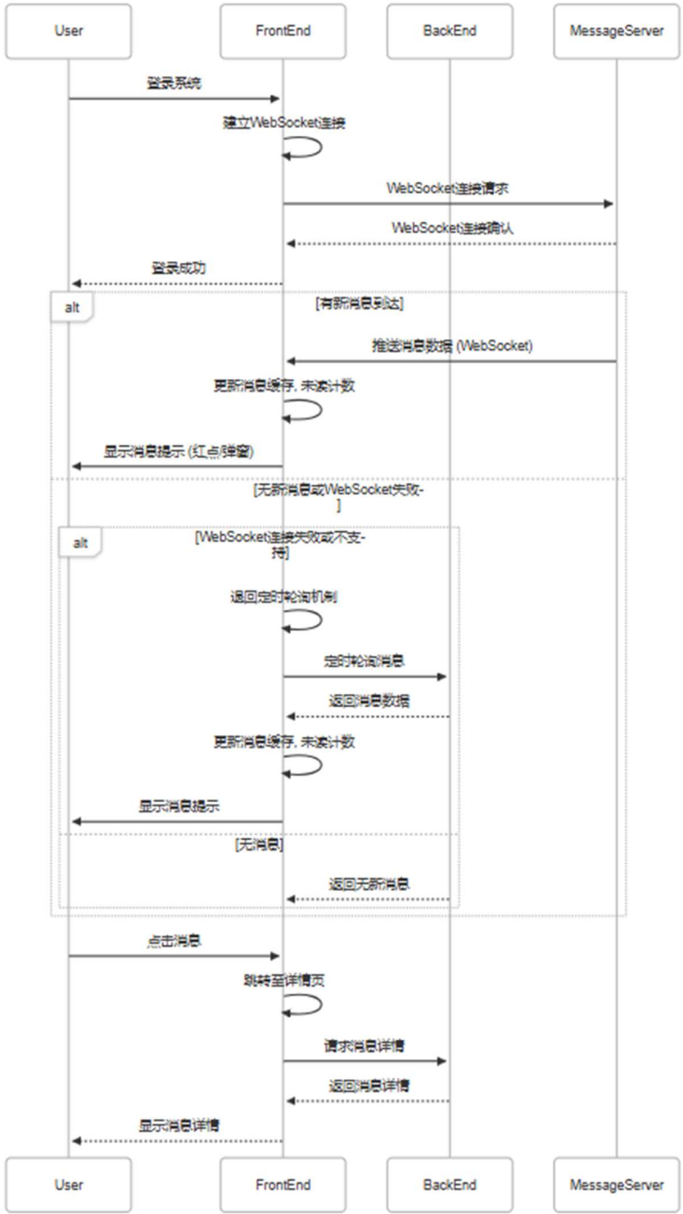
图 5：实时提醒功能顺序图
