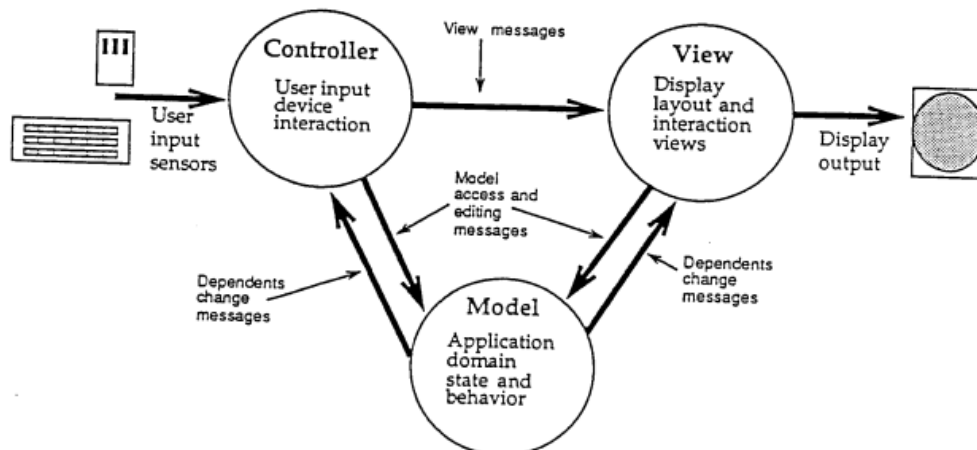
Figura 3: Representación del patrón MVC.
