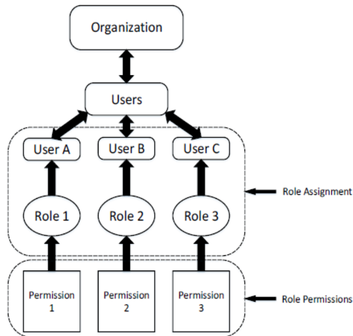
Figura 4: Representación del control de acceso basado en roles (RBAC).
