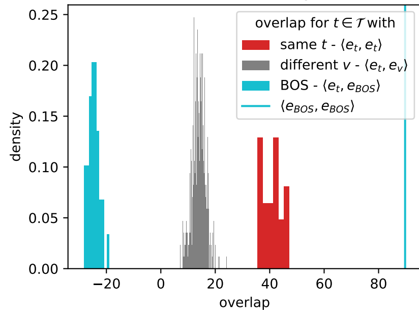
token embeddings
