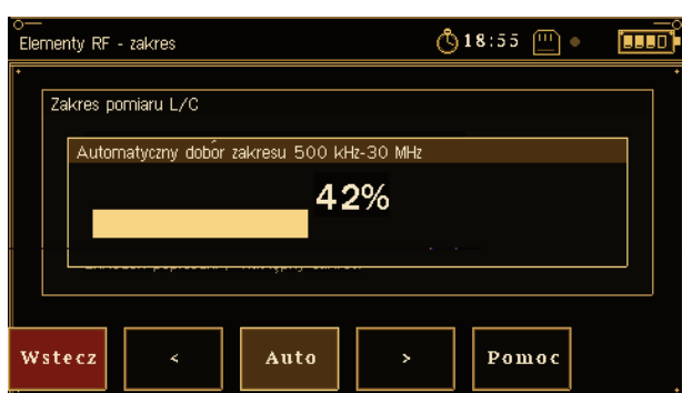
Rys. 5.4a. Skan automatyczny 500 kHz–30 MHz.
