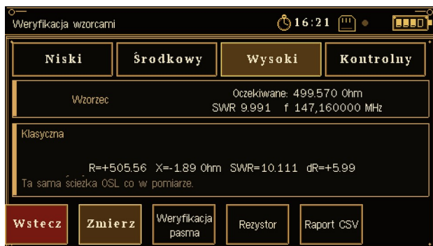
Rys. 1.15. Wzorec Wysoki: 499,570 \Omega . Przy 147,160 MHz analizator pokazał R=+505,56 \Omega , X=-1,89 \Omega i SWR=10,111 .
