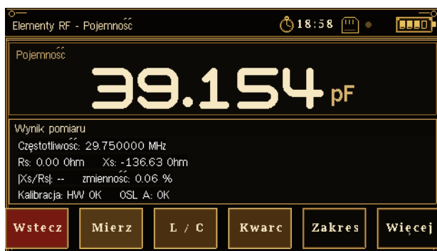
Rys. 5.5a. 39,154 pF przy 29,750 MHz.
