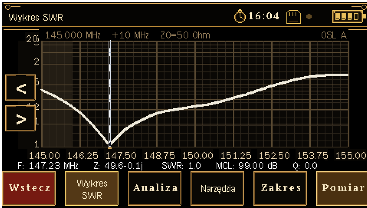
Rys. 2.11. Podstawowy widok SWR po zakończeniu skanu 145–155 MHz. Cursor znajduje się w pobliżu minimum: F 147,23 MHz, Z 49,6–0,1j \Omega , SWR 1,0, MCL 99,00 dB, Q 0,0. Aktualnie użyta korekcja jest oznaczona jako OSL A.
