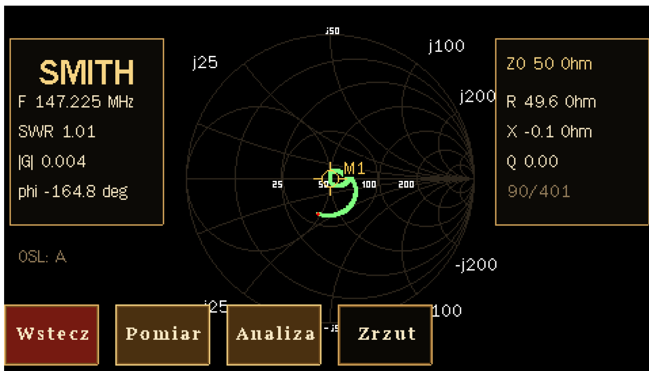
Rys. 2.26. Pełny Smith wywołany z bieżącego skanu. Dla punktu 147,225 MHz: SWR 1,01, |\Gamma| 0,004, faza \Gamma -164,8°, R 49,6 \Omega , X -0,1 \Omega , punkt 90/401, OSL A.
