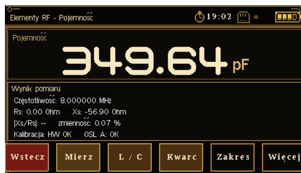
Rys. 5.5b. 349,64 pF przy 8,000 MHz.
