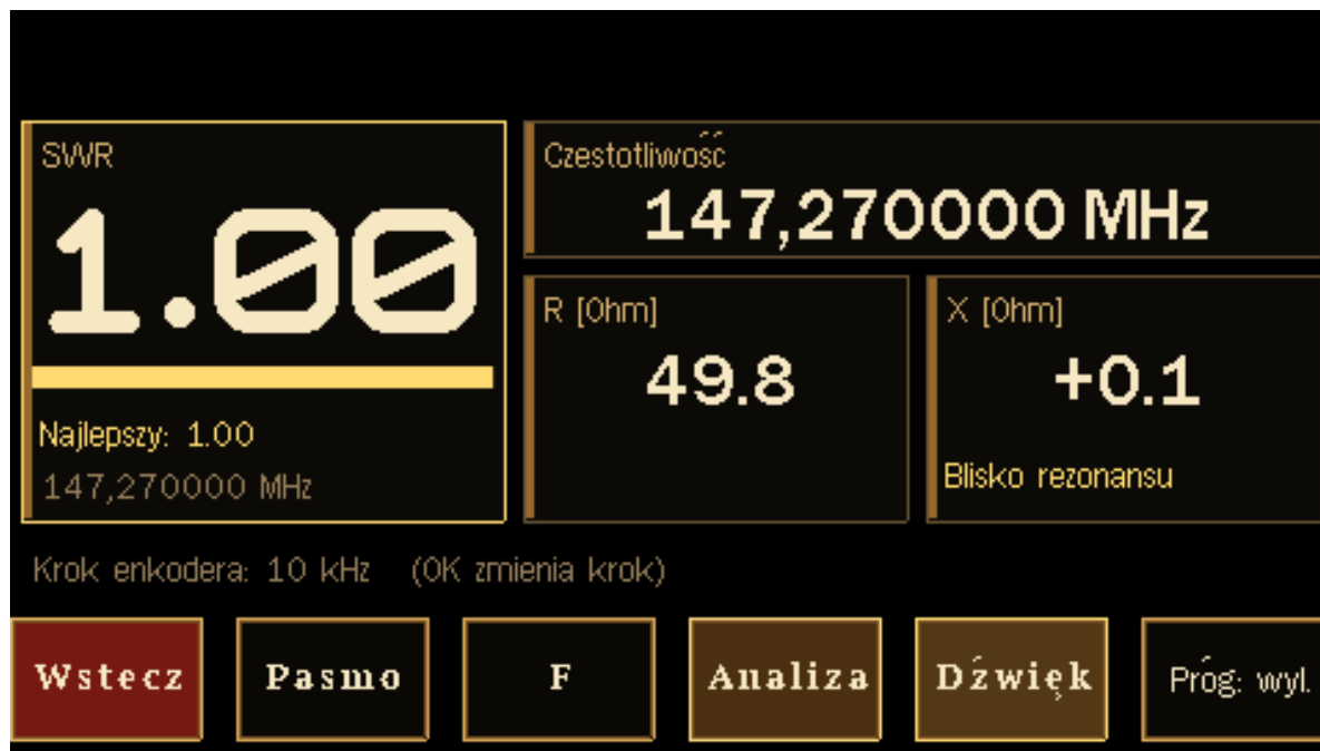
Rys. 4.10. Pomiar ciągły w pobliżu najlepszego punktu: 147,270 MHz, SWR 1,00, R \approx 49,8 \Omega i X \approx +0,1 \Omega .
