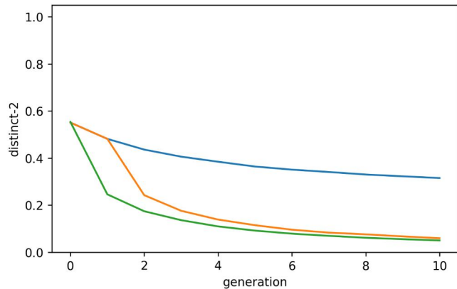
D. Distinct-2
