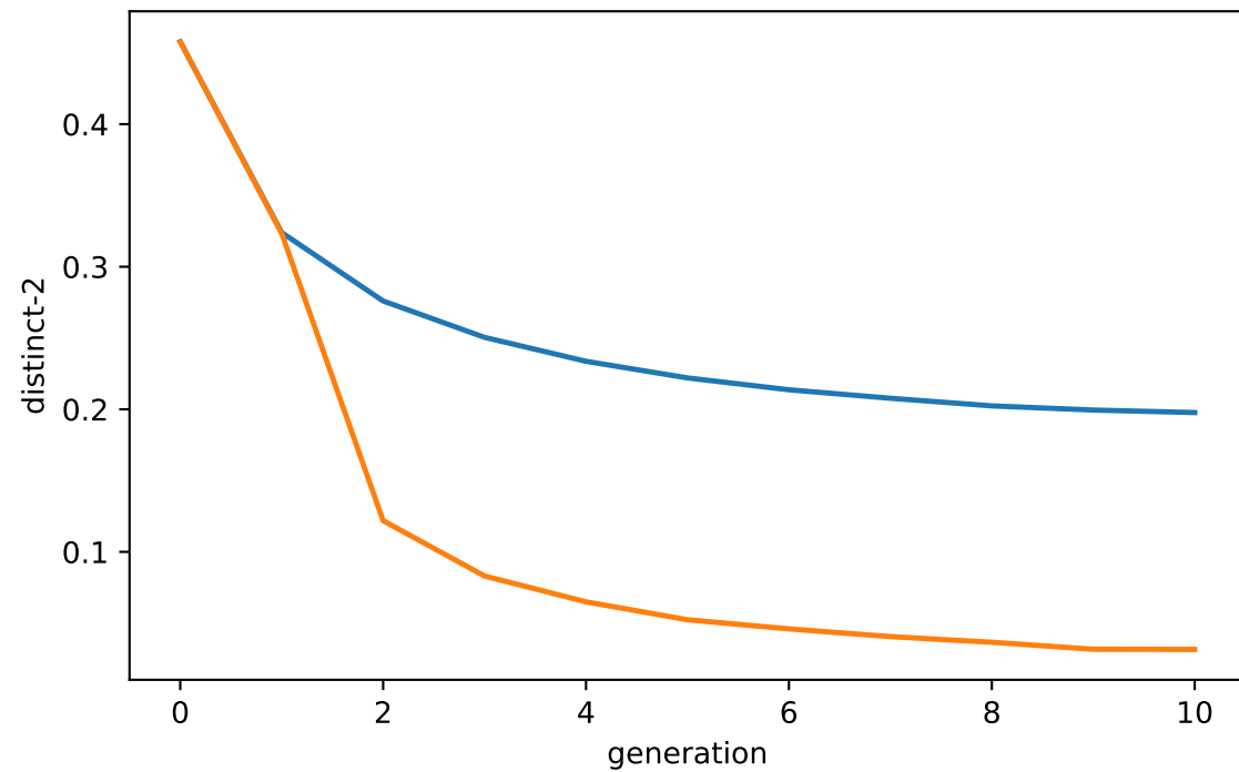
D. Distinct-2
