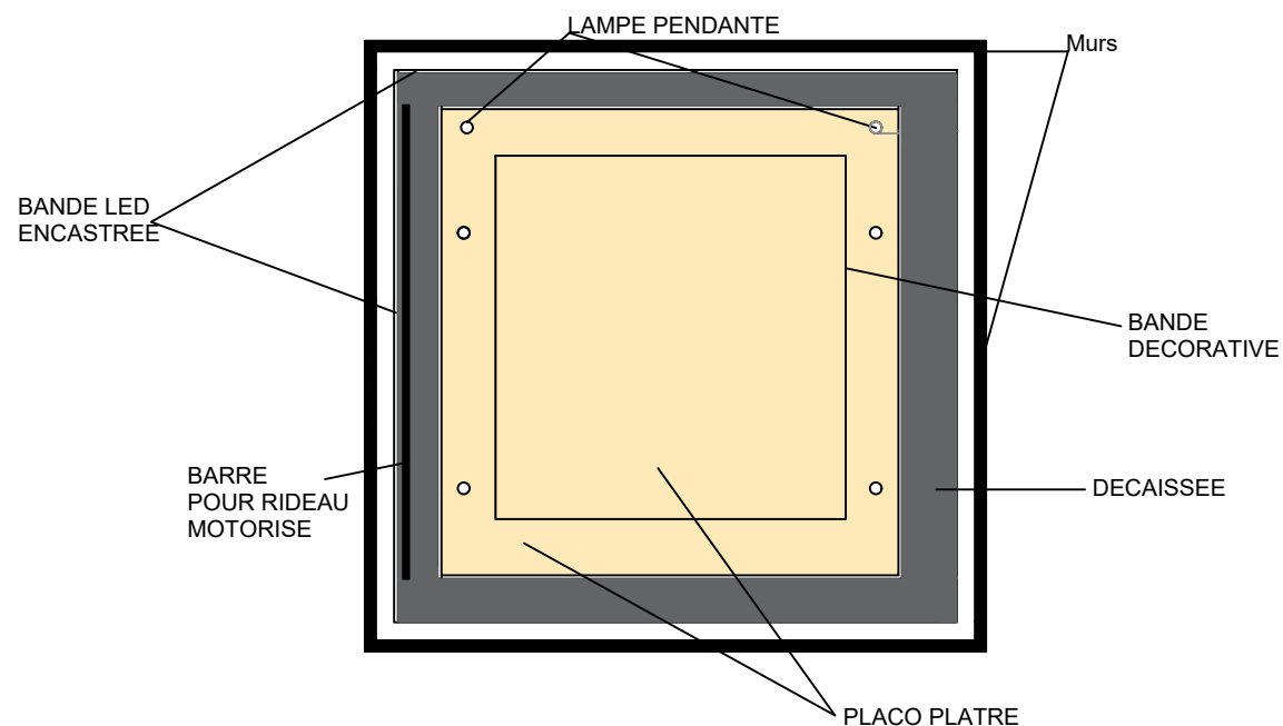
PLAFOND CHAMBRES ENFANTS
