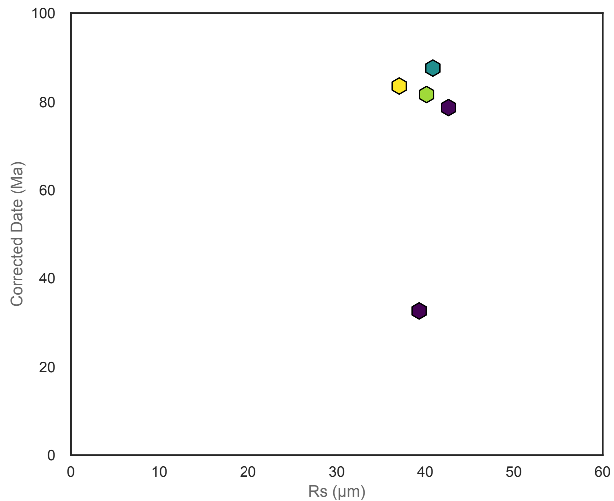
Sample AN3-06 - AHe
