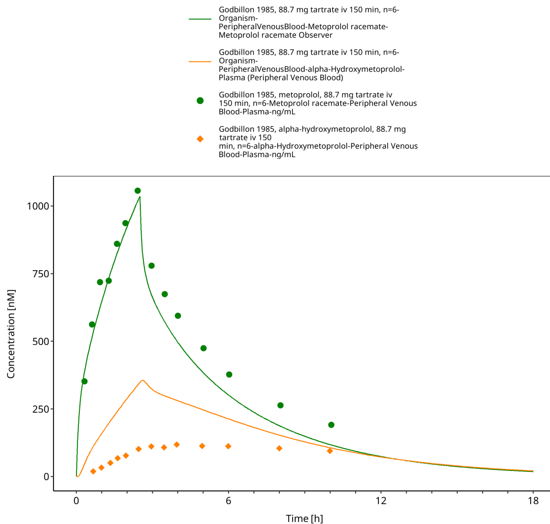
Figure 3-29: Godbillon 1985: 88.7 mg tartrate iv 150 min, n=6
