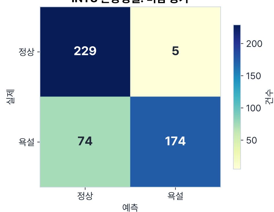
INT8 혼동행렬: 미탐 증가
