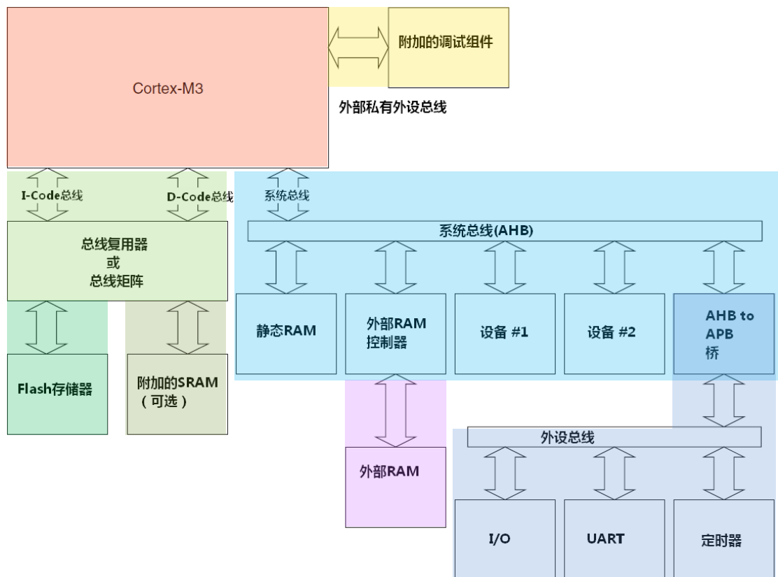
图 6.4 Cortex-M3 总线连接范例
