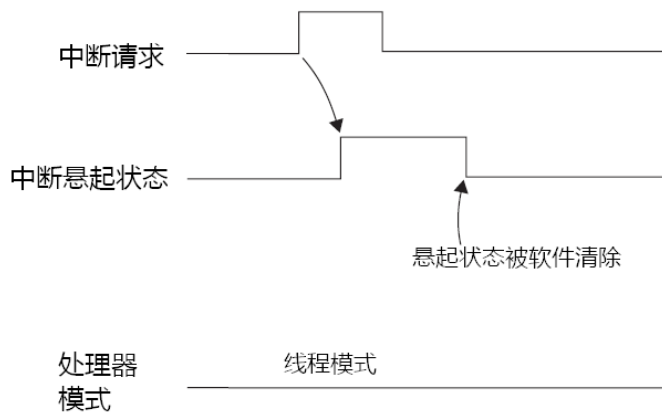
图 7.9 中断在得到处理器响应之前被清除悬起状态
