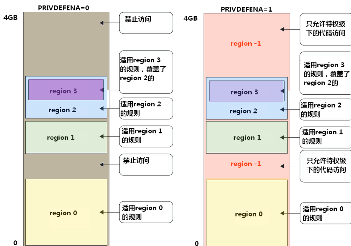
图14.1 PRIVDEFENA的影响
