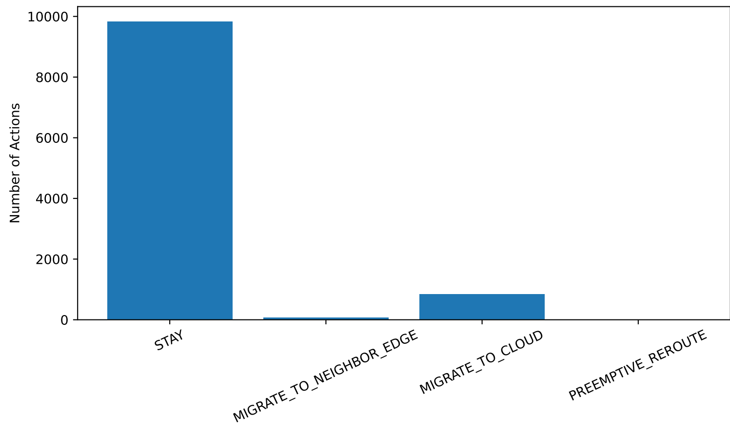
MAPPO Action Distribution
