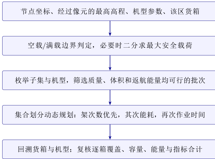
图 5 单点运输能力与货箱组批求解流程
