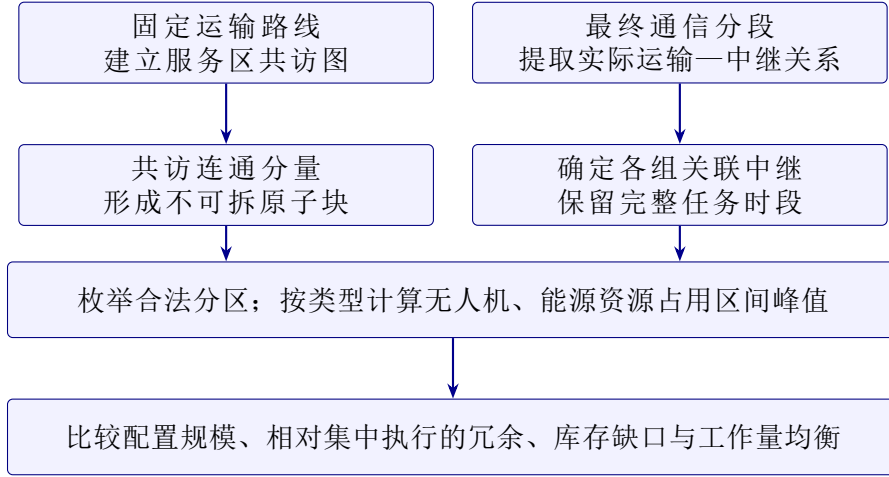
图 12 固定方案分区与资源核算流程；不代表已求得的具体服务区分组
