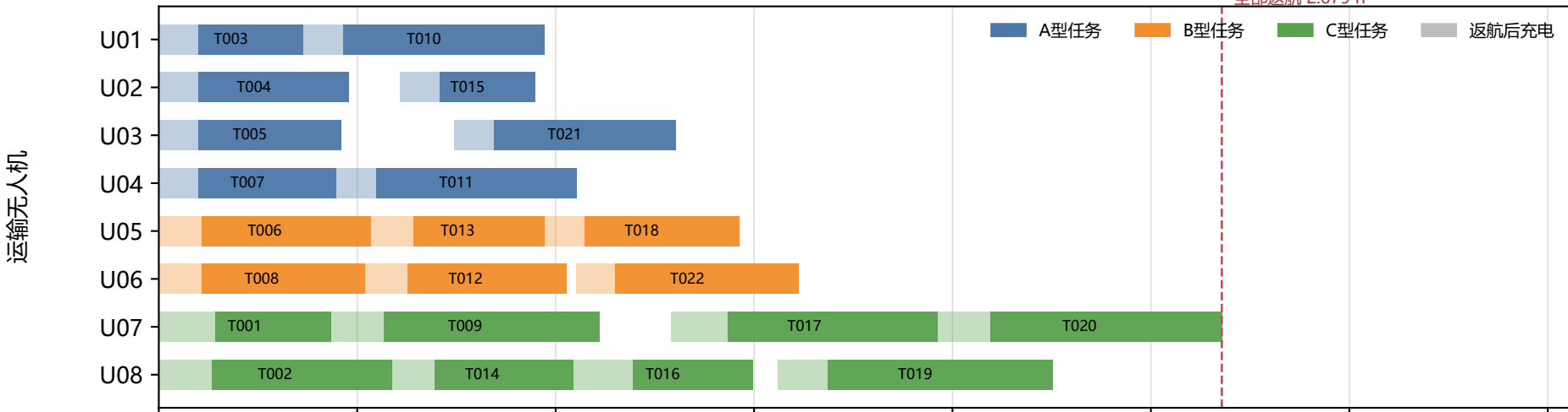
(a) 实体运输无人机占用
