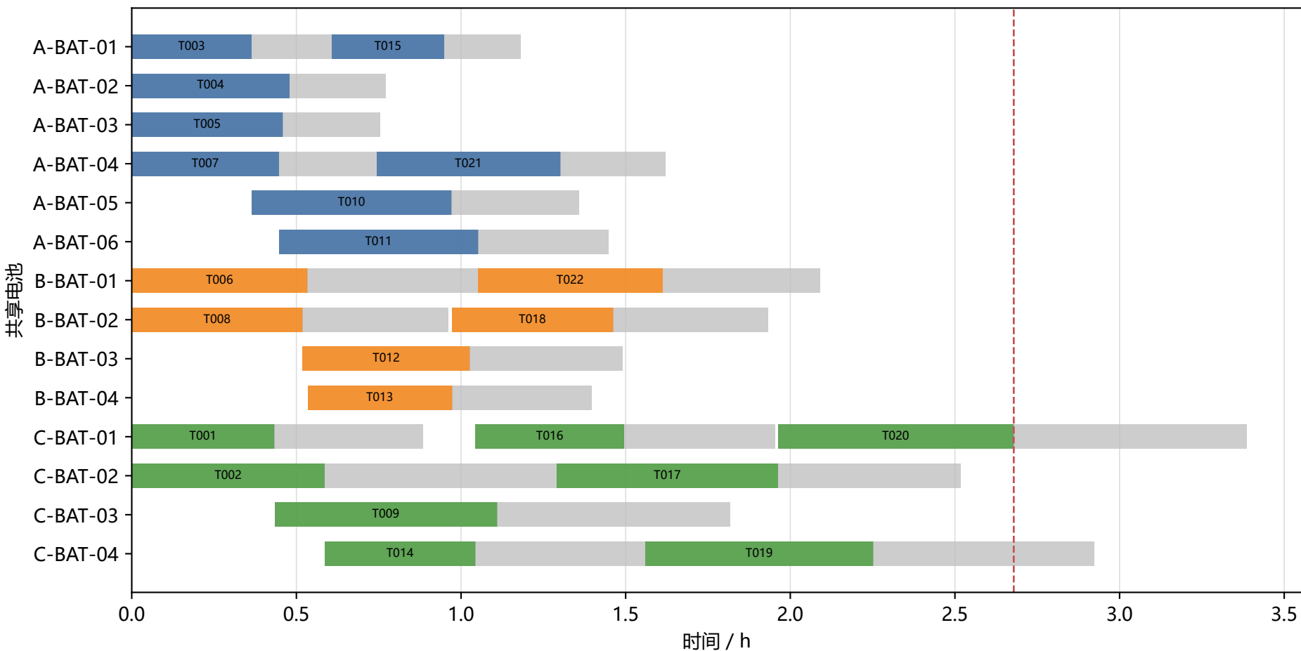
(b) 共享电池任务与充电占用
