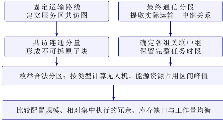
图 15 固定方案分区与资源核算流程；不代表已求得的具体服务区分组
