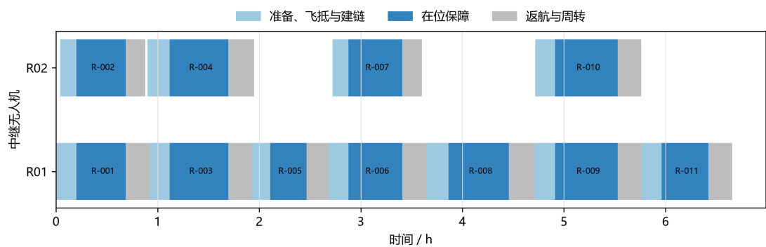
图 12 中继波次与实体资源占用时间轴
