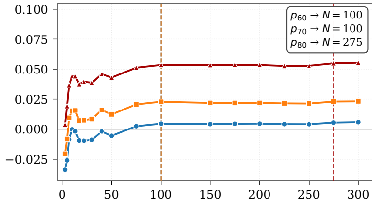
SuperDialseg
