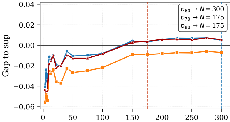
TIAGE
