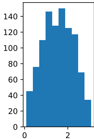
inclination
