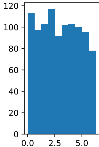
ra
