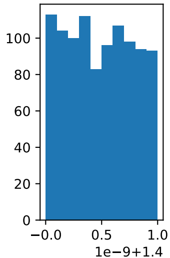
ra
