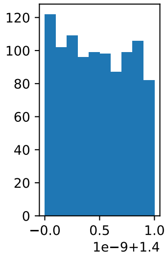
inclination
