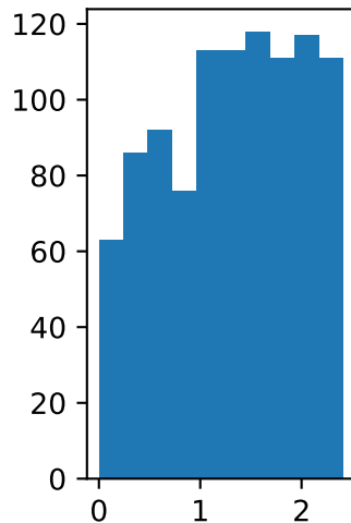
redshift
