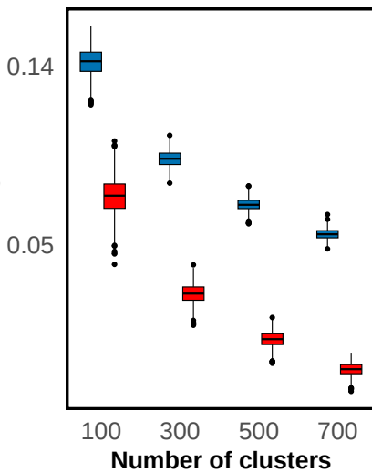
CI Length
