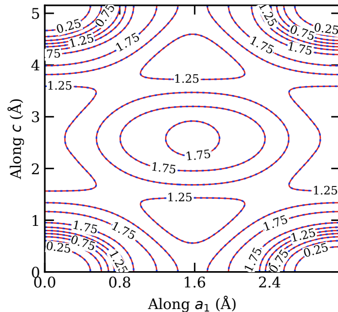
(d) Mg (011̄0)
