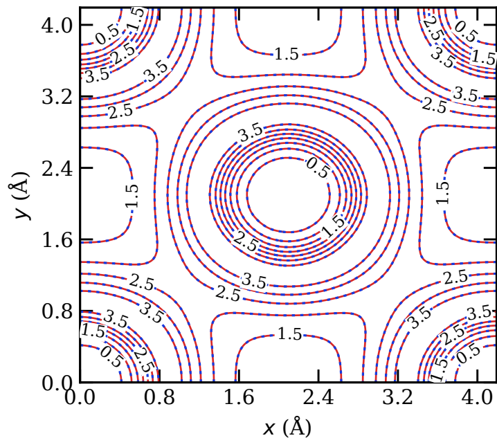
(a) Al (001)
