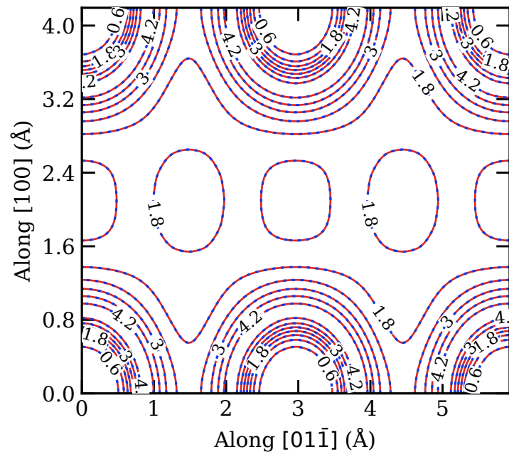
(b) Al (011)
